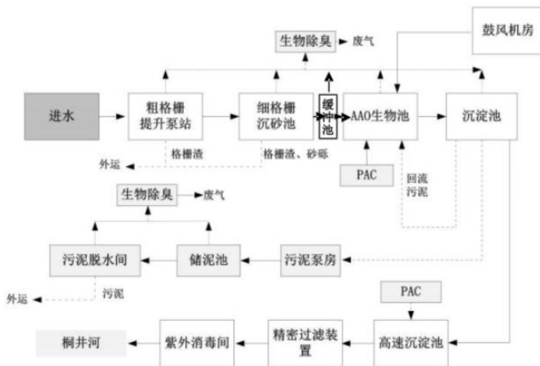
图 6.3-2 棠下污水处理厂一期工程污水处理工艺
