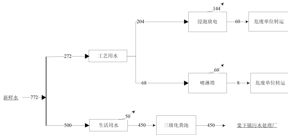
图 3.2-2 项目水平衡图 （单位：吨/年）
