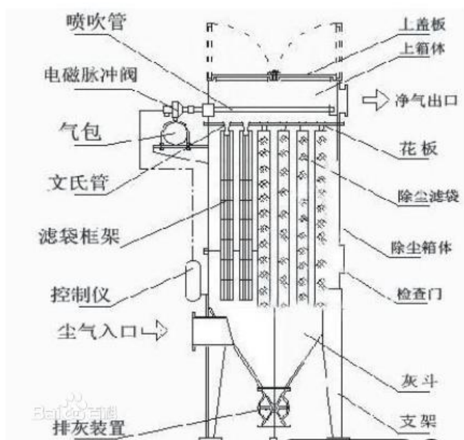
脉冲布袋除尘器构造图
