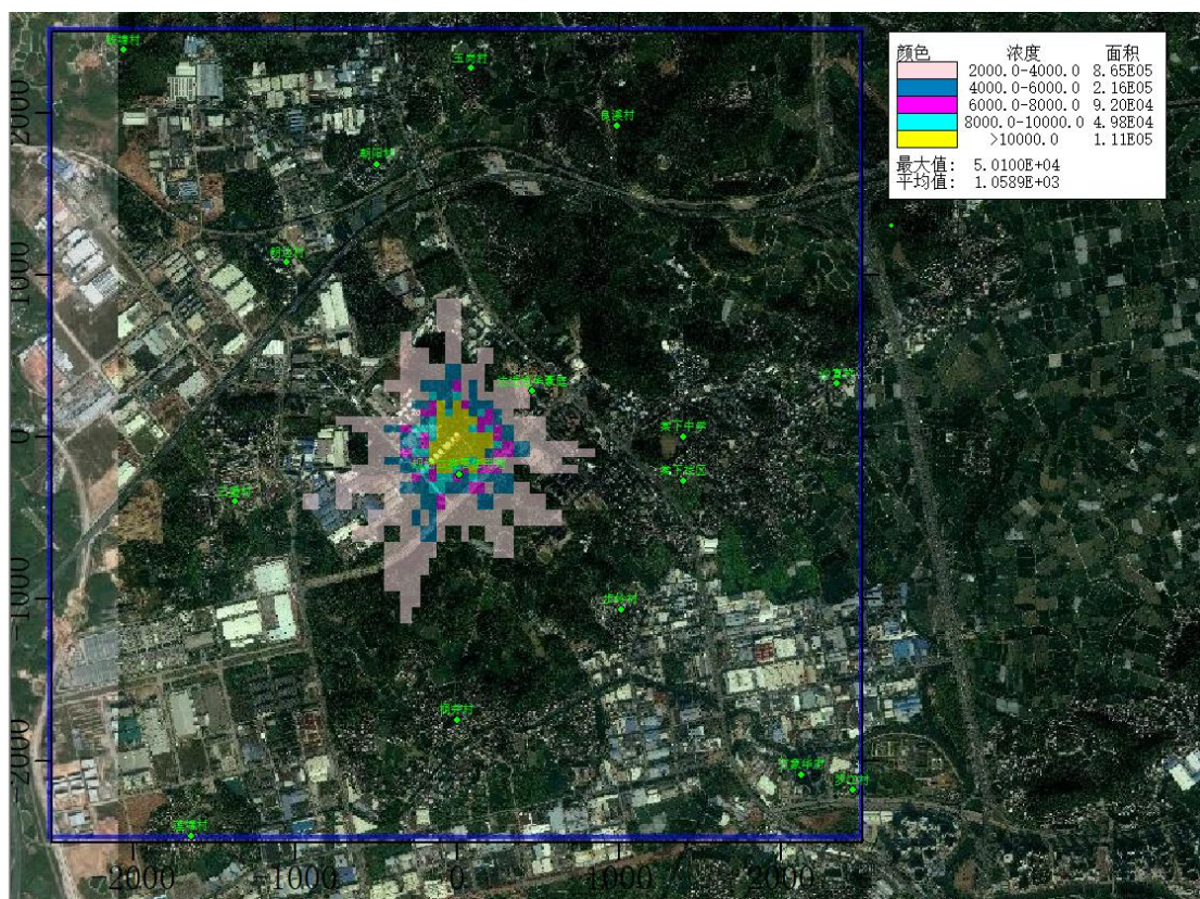
图 5.4.2.2-49 非正常工况下非甲烷总烃小时贡献值等值线图（浓度单位 \mu\text{g}/\text{m}^3 ）
