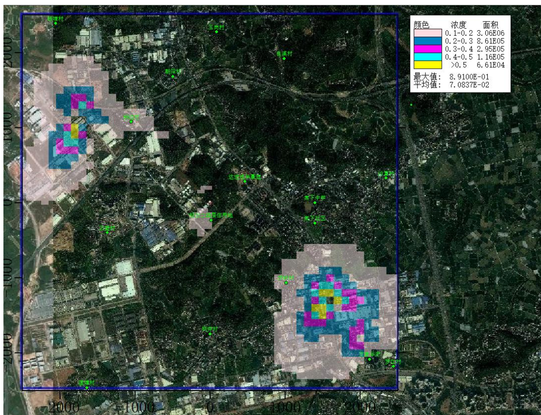
图 5.4.2.2-27 建成后叠加背景值后 PM 10 年平均浓度等值线图（浓度单位 \mu\text{g}/\text{m}^3 ）
