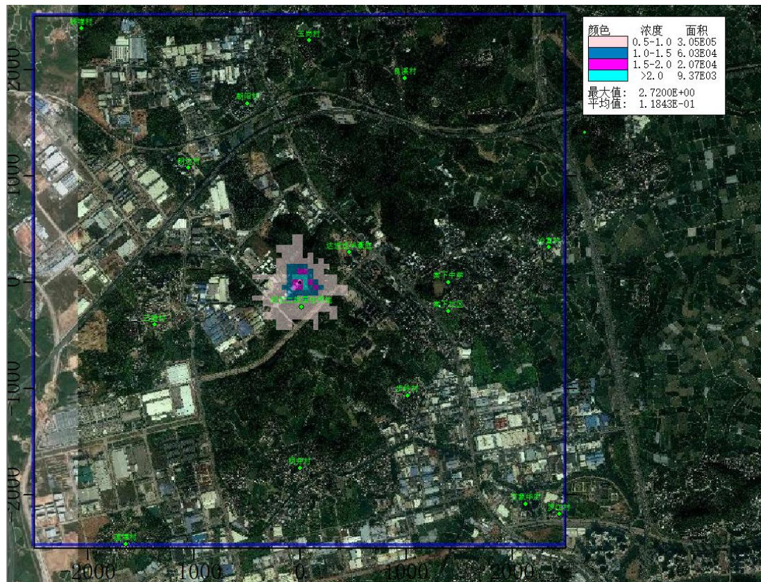
图 5.4.2.2-31 建成后叠加背景值后氟化物小时浓度等值线图（浓度单位 \mu\text{g}/\text{m}^3 ）
