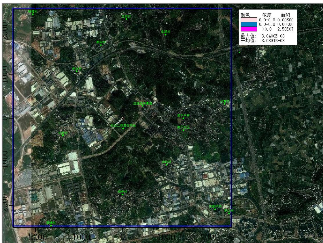
图 5.4.2.2-47 建成后叠加背景值后二噁英年平均浓度等值线图（浓度单位 \mu\text{g}/\text{m}^3 ）
