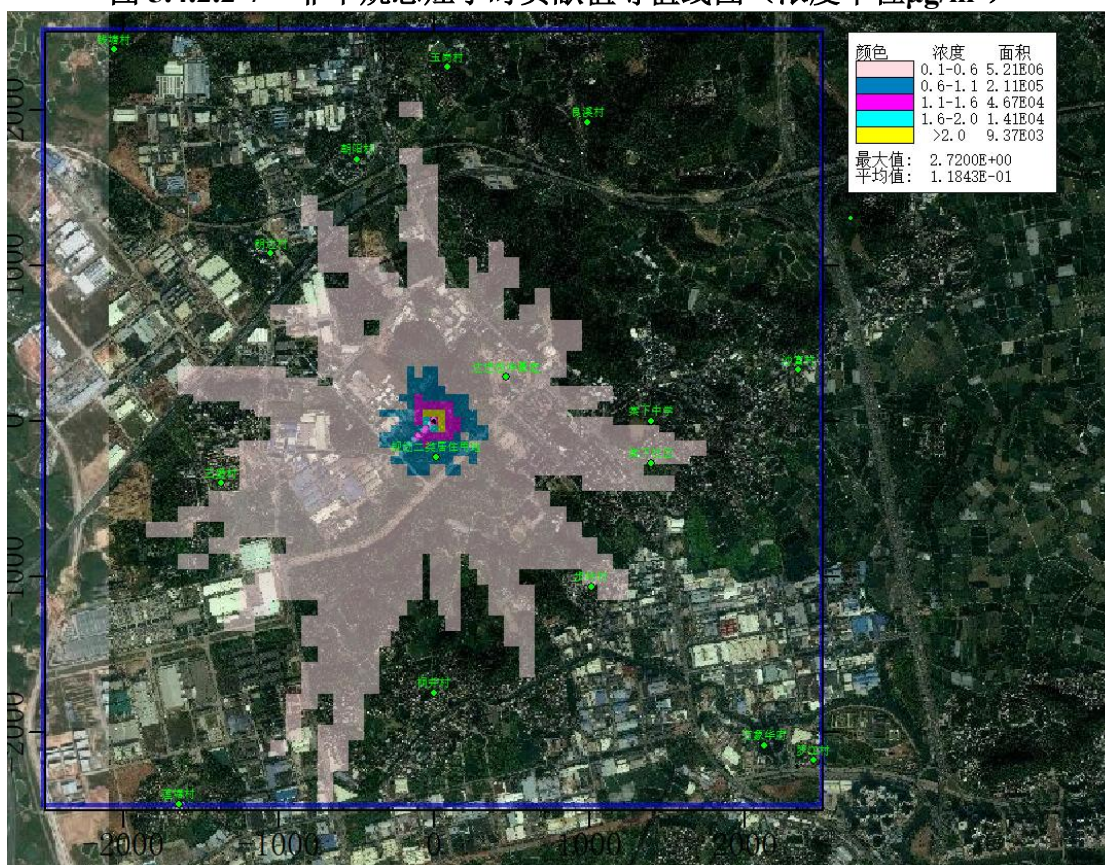
图 5.4.2.2-8 氟化物小时贡献值等值线图（浓度单位 \mu\text{g}/\text{m}^3 ）
