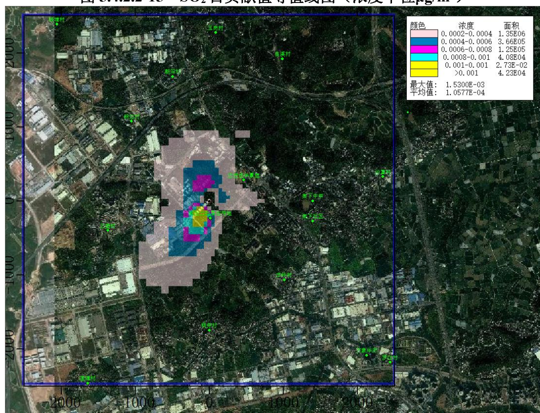
图 5.4.2.2-16 SO 2 年贡献值等值线图（浓度单位 \mu\text{g}/\text{m}^3 ）
