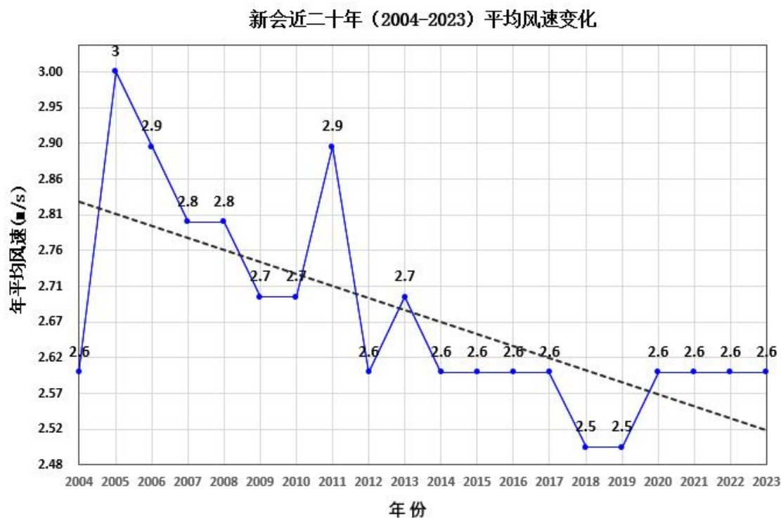
图 4.1.5-3 新会气象站近 20 年(2004~2023 年)年平均风速
