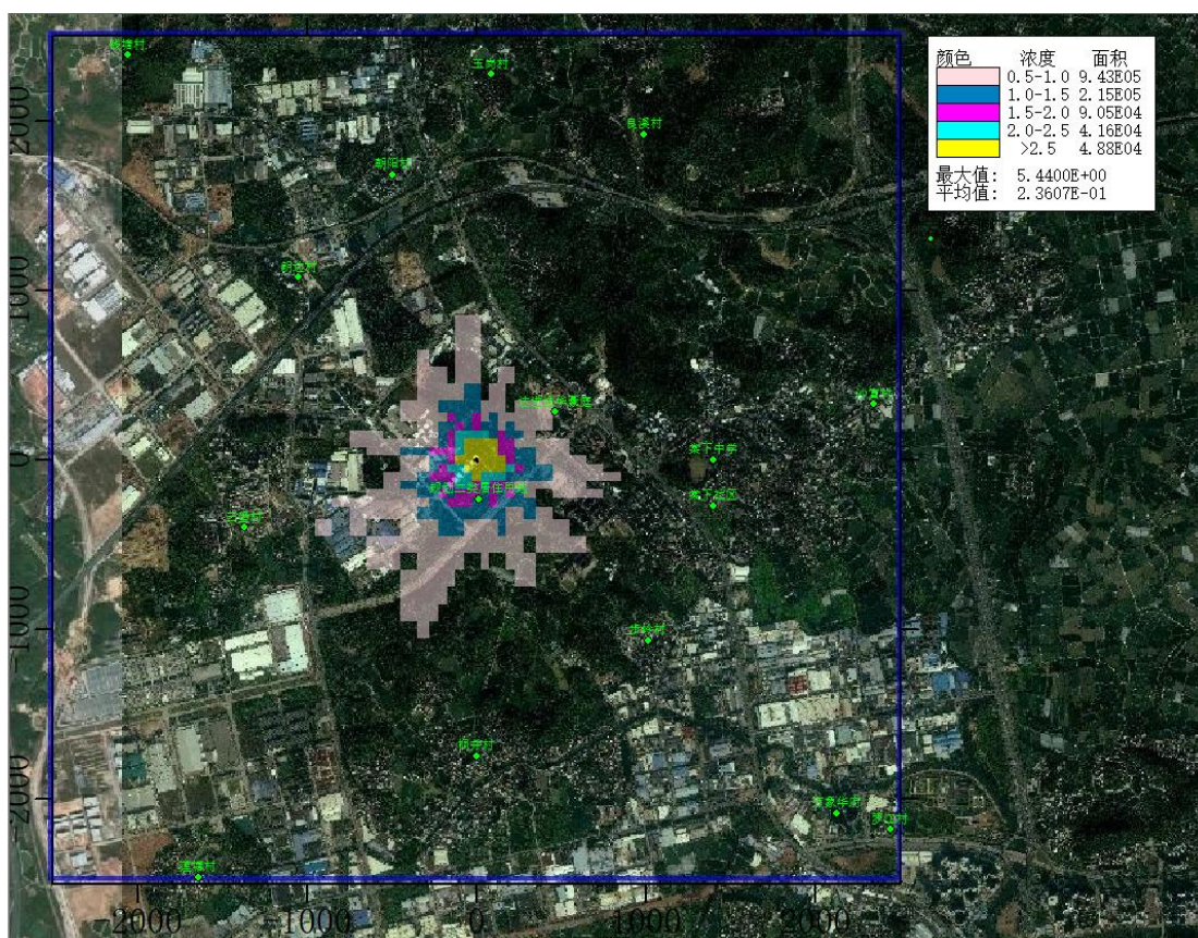
图 5.4.2.2-10 镍及其化合物小时平均贡献值等值线图（浓度单位 \mu\text{g}/\text{m}^3 ）
