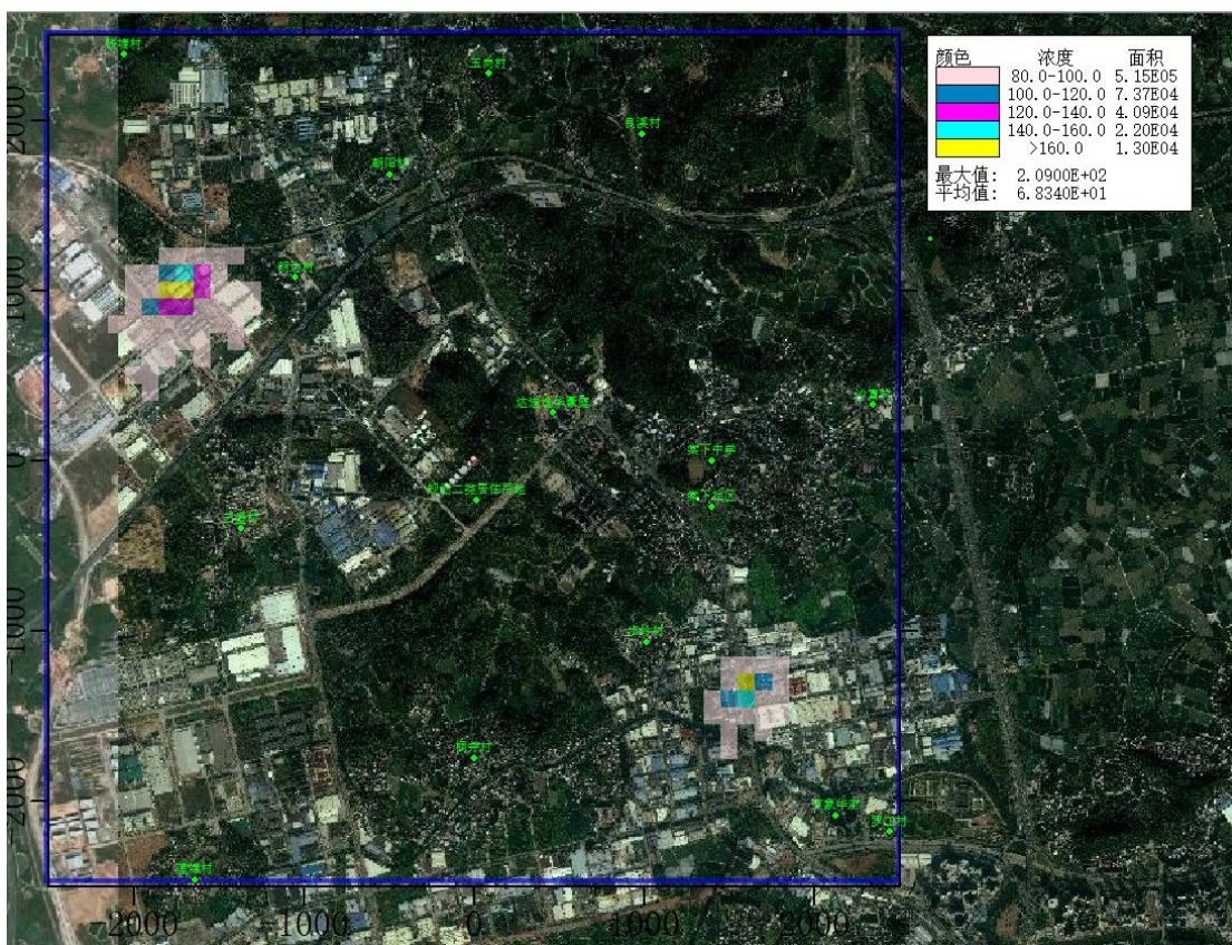
图 5.4.2.2-28 建成后叠加背景值后 TSP 日平均浓度等值线图（浓度单位 \mu\text{g}/\text{m}^3 ）
