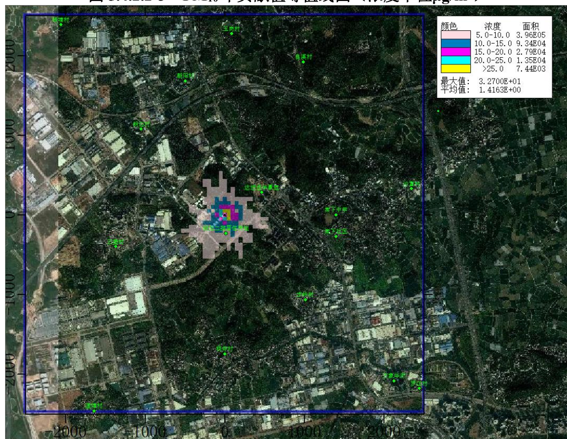
图 5.4.2.2-4 TSP 小时贡献值等值线图（浓度单位 \mu\text{g}/\text{m}^3 ）
