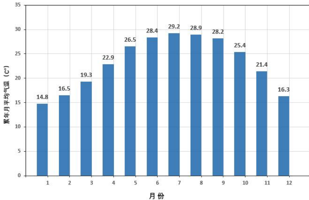
图 4.1.5-4 新会气象站近 20 年(2004~2023 年)月平均气温
