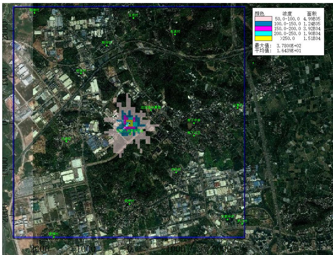
图 5.4.2.2-23 TVOC 小时贡献值等值线图（浓度单位 \mu\text{g}/\text{m}^3 ）
