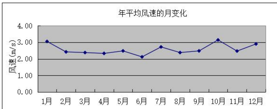
图 4.1.5-13 平均风速的月变化曲线图
