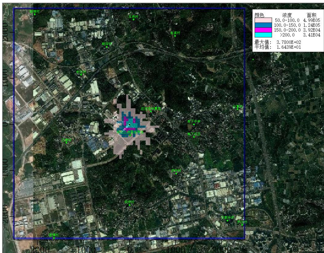
图 5.4.2.2-7 非甲烷总烃小时贡献值等值线图（浓度单位 \mu\text{g}/\text{m}^3 ）
