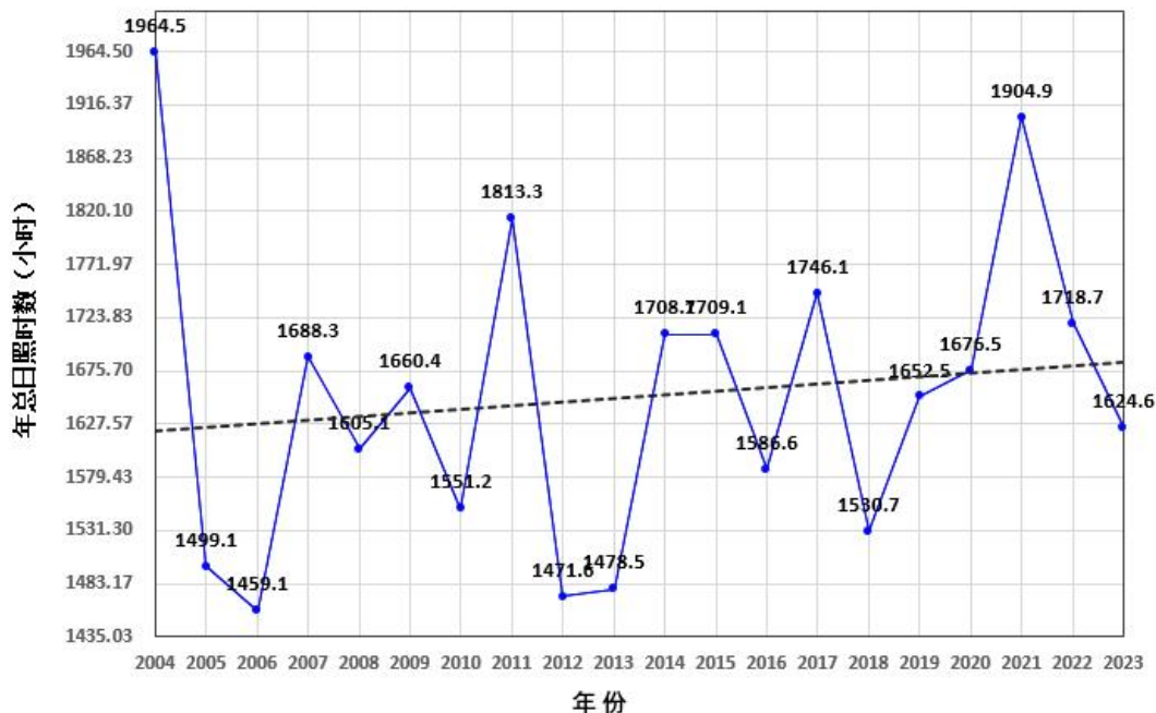
图 4.1.5-9 新会气象站近 20 年(2004~2023 年)年平均日照
