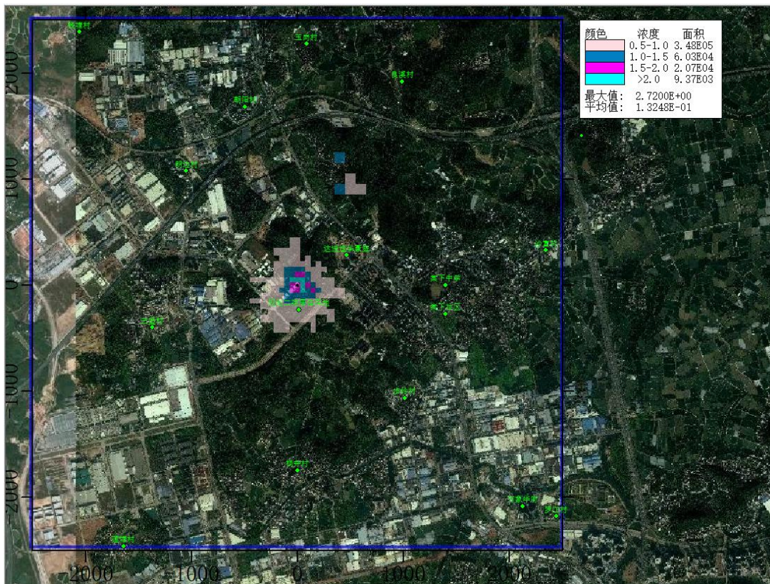
图 5.4.2.2-34 建成后叠加背景值后锰及其化合物小时浓度等值线图（浓度单位 \mu\text{g}/\text{m}^3 ）
