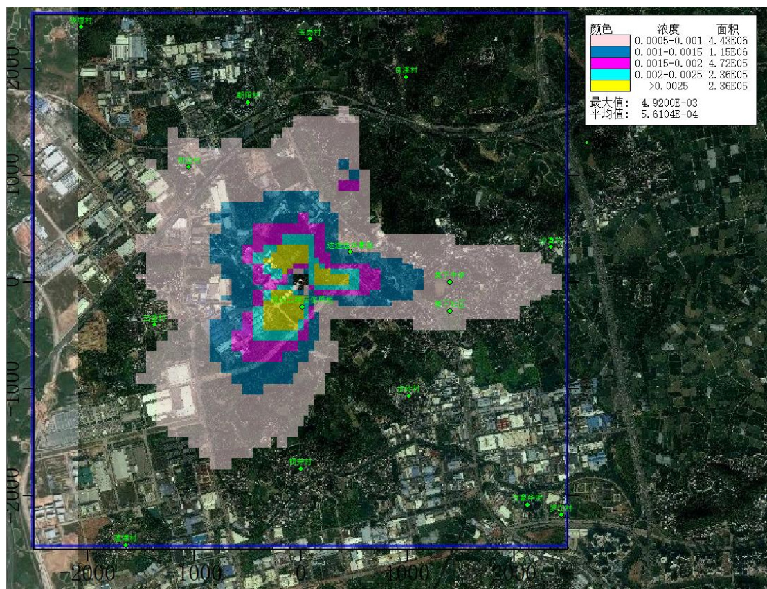
图 5.4.2.2-15 SO 2 日贡献值等值线图（浓度单位 \mu\text{g}/\text{m}^3 ）
