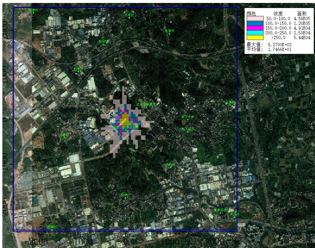
图 5.4.2.2-53 非正常工况下钴及其化合物小时贡献值等值线图（浓度单位 \mu\text{g}/\text{m}^3 ）
