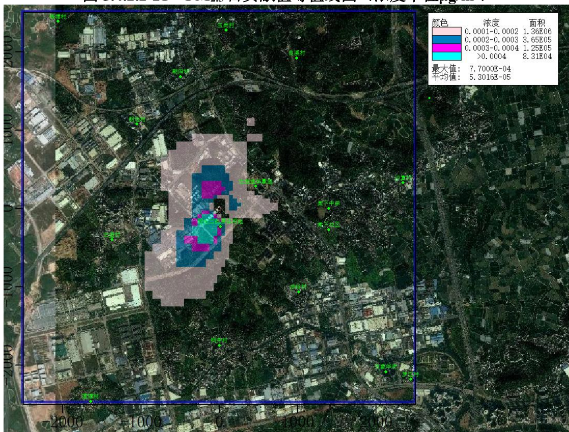
图 5.4.2.2-22 PM 2.5 年贡献值等值线图（浓度单位 \mu\text{g}/\text{m}^3 ）
