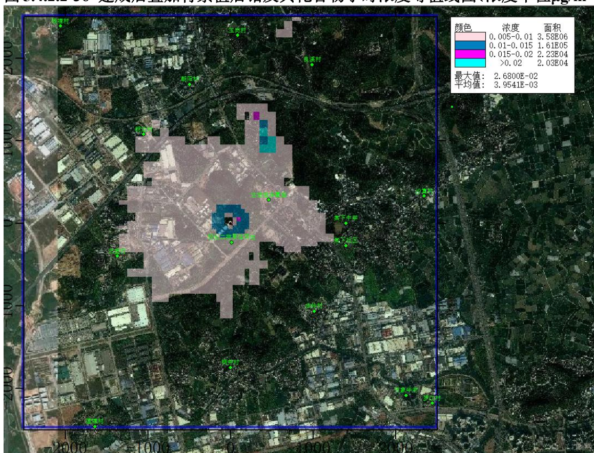
图 5.4.2.2-37 建成后叠加背景值后 \text{SO}_2 小时浓度等值线图 (浓度单位 \mu\text{g}/\text{m}^3 )
