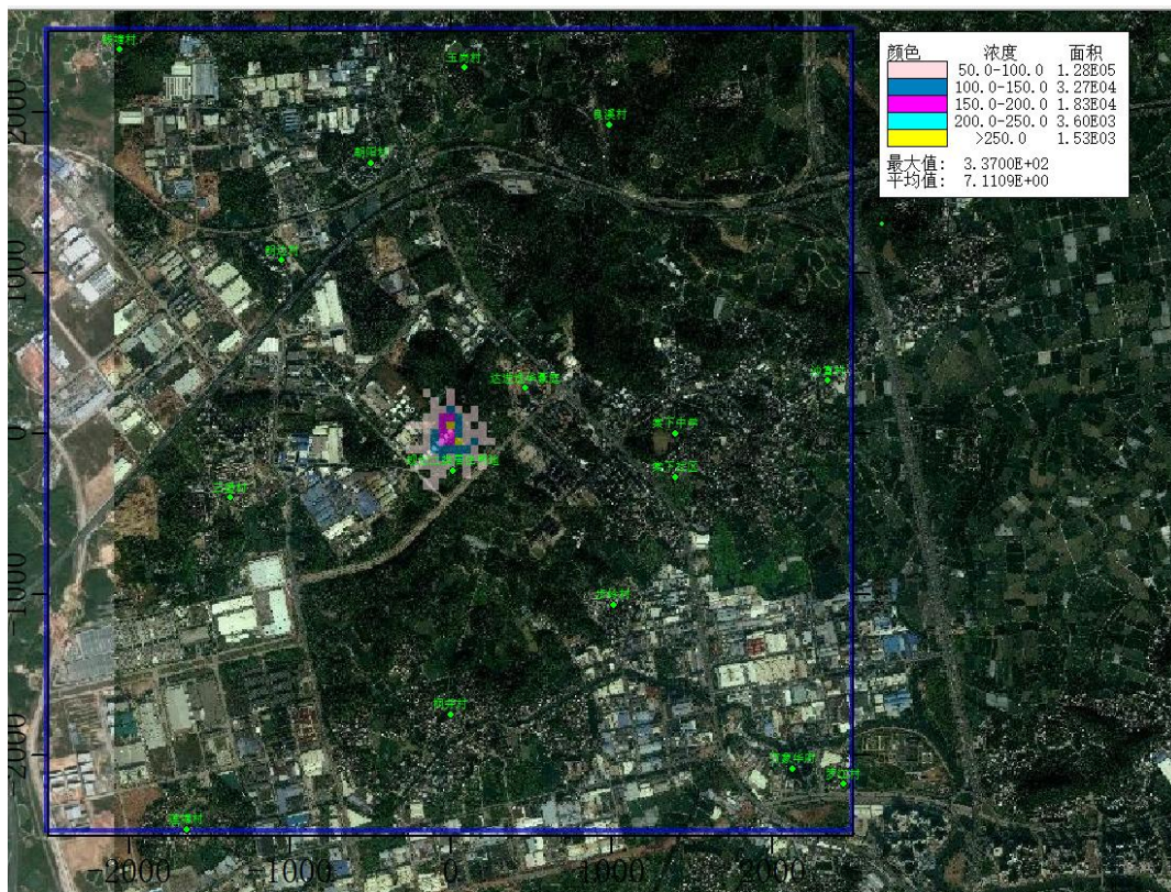
图 5.4.2.2-50 非正常工况下氟化物小时贡献值等值线图（浓度单位 \mu\text{g}/\text{m}^3 ）
