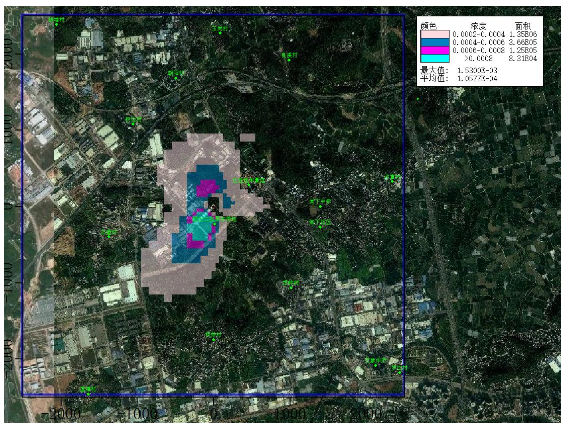
图 5.4.2.2-39 建成后叠加背景值后 SO 2 年平均浓度等值线图（浓度单位 μg/m 3 ）
