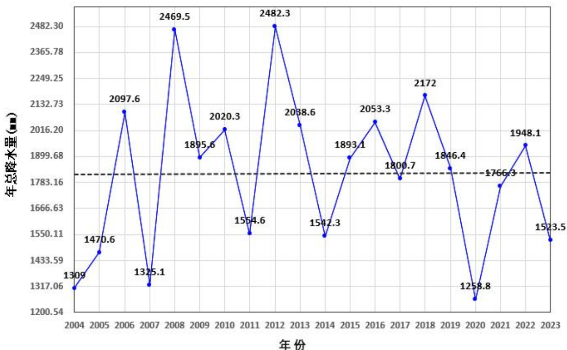
图 4.1.5-7 新会气象站近 20 年(2004~2023 年)年平均降水量
