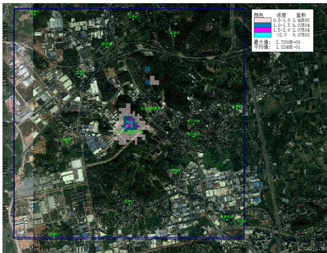
图 5.4.2.2-11 锰及其化合物小时平均贡献值等值线图（浓度单位 \mu\text{g}/\text{m}^3 ）
