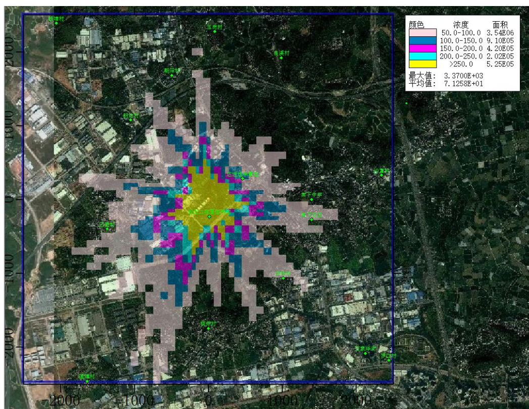
图 5.4.2.2-51 非正常工况下镍及其化合物小时贡献值等值线图（浓度单位 \mu\text{g}/\text{m}^3 ）
