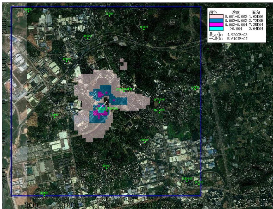
图 5.4.2.2-38 建成后叠加背景值后 SO 2 日平均浓度等值线图（浓度单位 μg/m 3 ）
