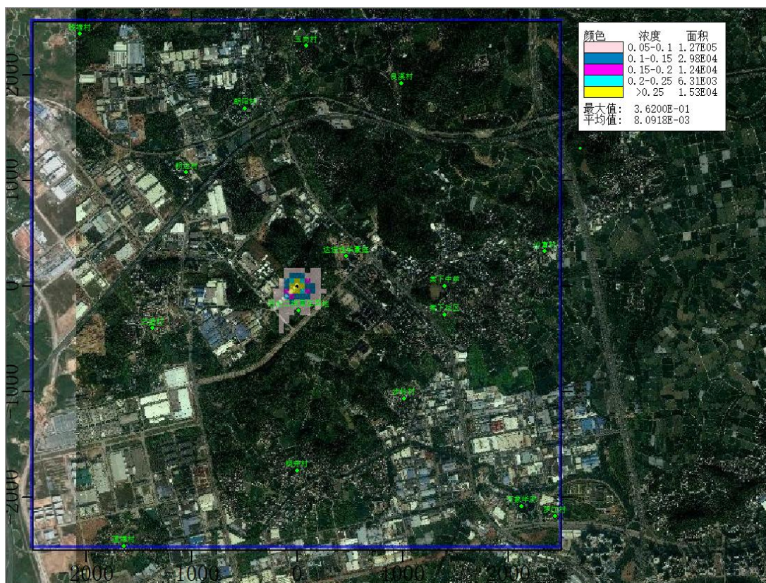
图 5.4.2.2-32 建成后叠加背景值后氟化物日均浓度等值线图（浓度单位 \mu\text{g}/\text{m}^3 ）
