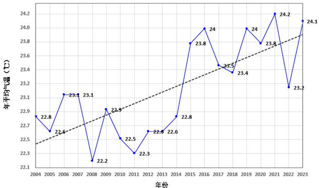
图 4.1.5-5 新会气象站近 20 年(2004~2023 年)年平均气温
