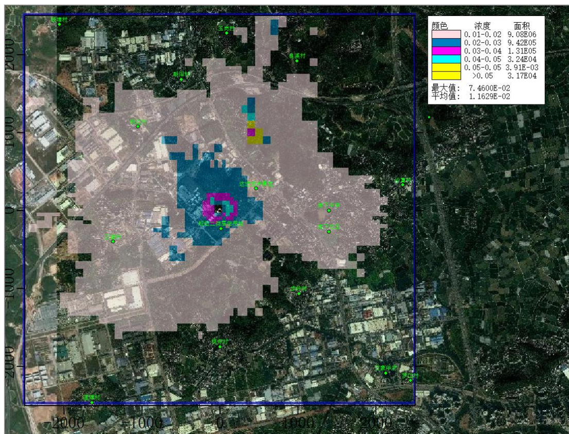
图 5.4.2.2-17 NO 2 小时贡献值等值线图（浓度单位 \mu\text{g}/\text{m}^3 ）
