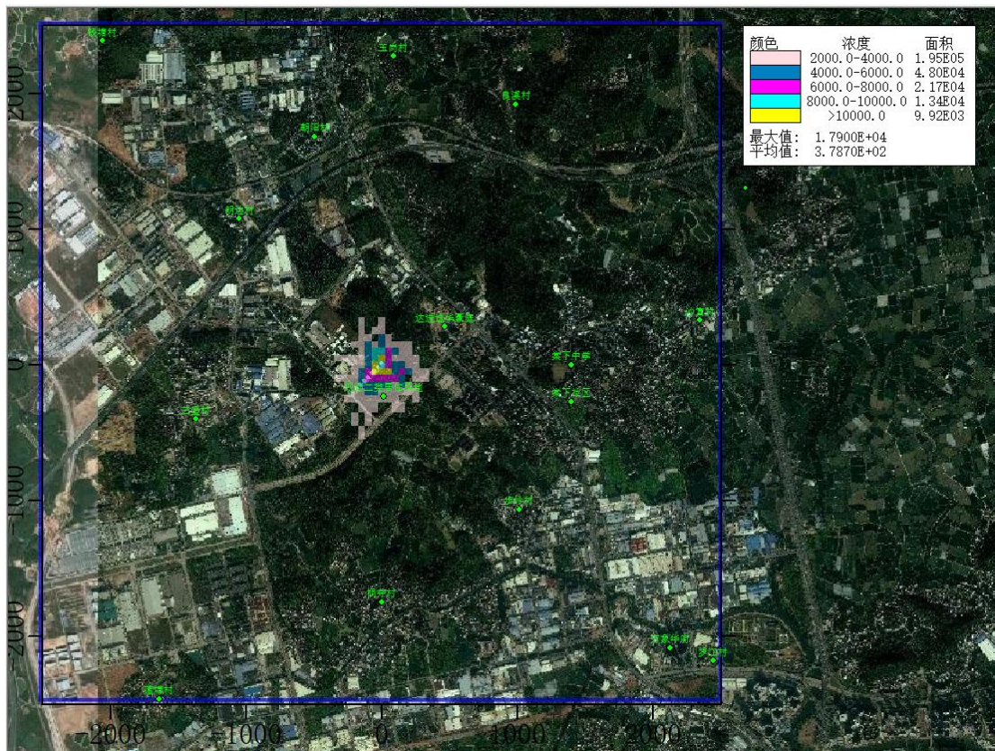
图 5.4.2.2-48 非正常工况下 TSP 小时贡献值等值线图（浓度单位 \mu\text{g}/\text{m}^3 ）
