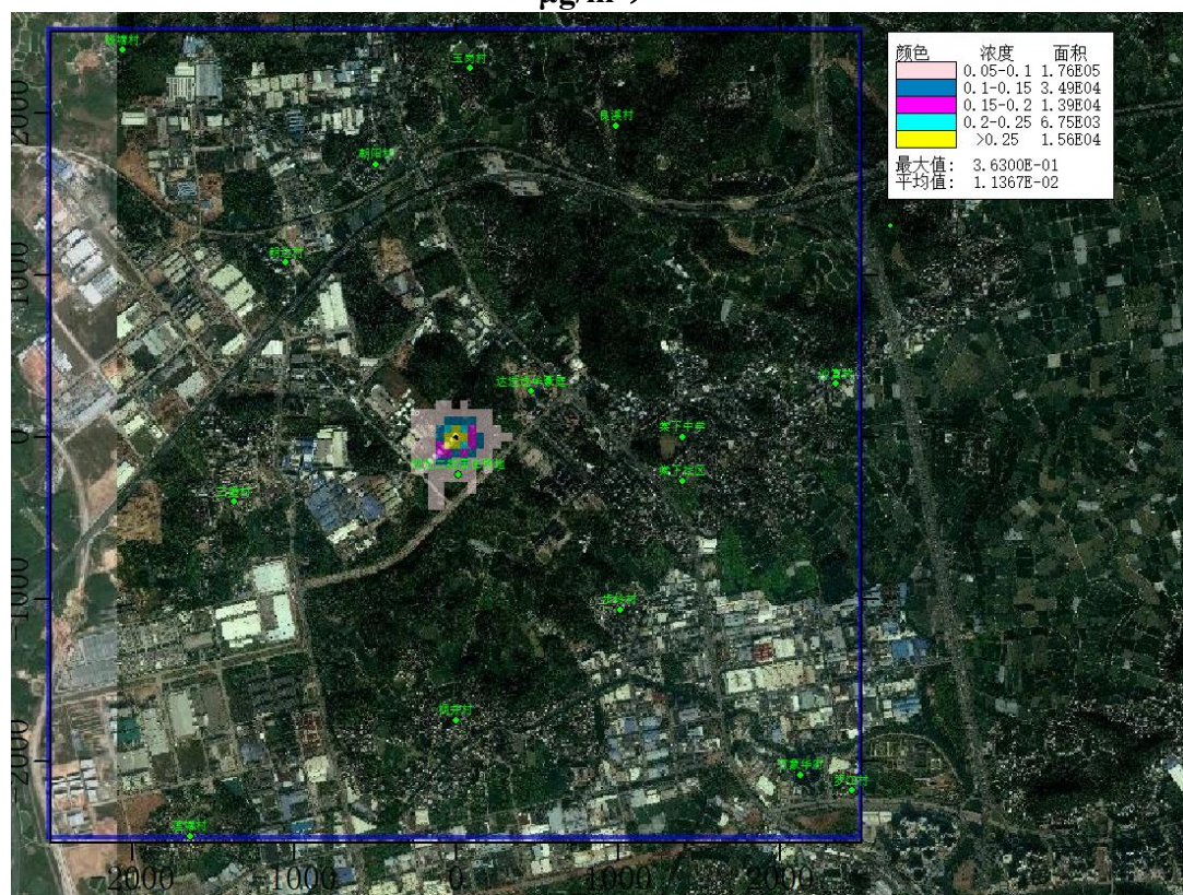
图 5.4.2.2-35 建成后叠加背景值后锰及其化合物日均浓度等值线图（浓度单位 \mu\text{g}/\text{m}^3 ）
