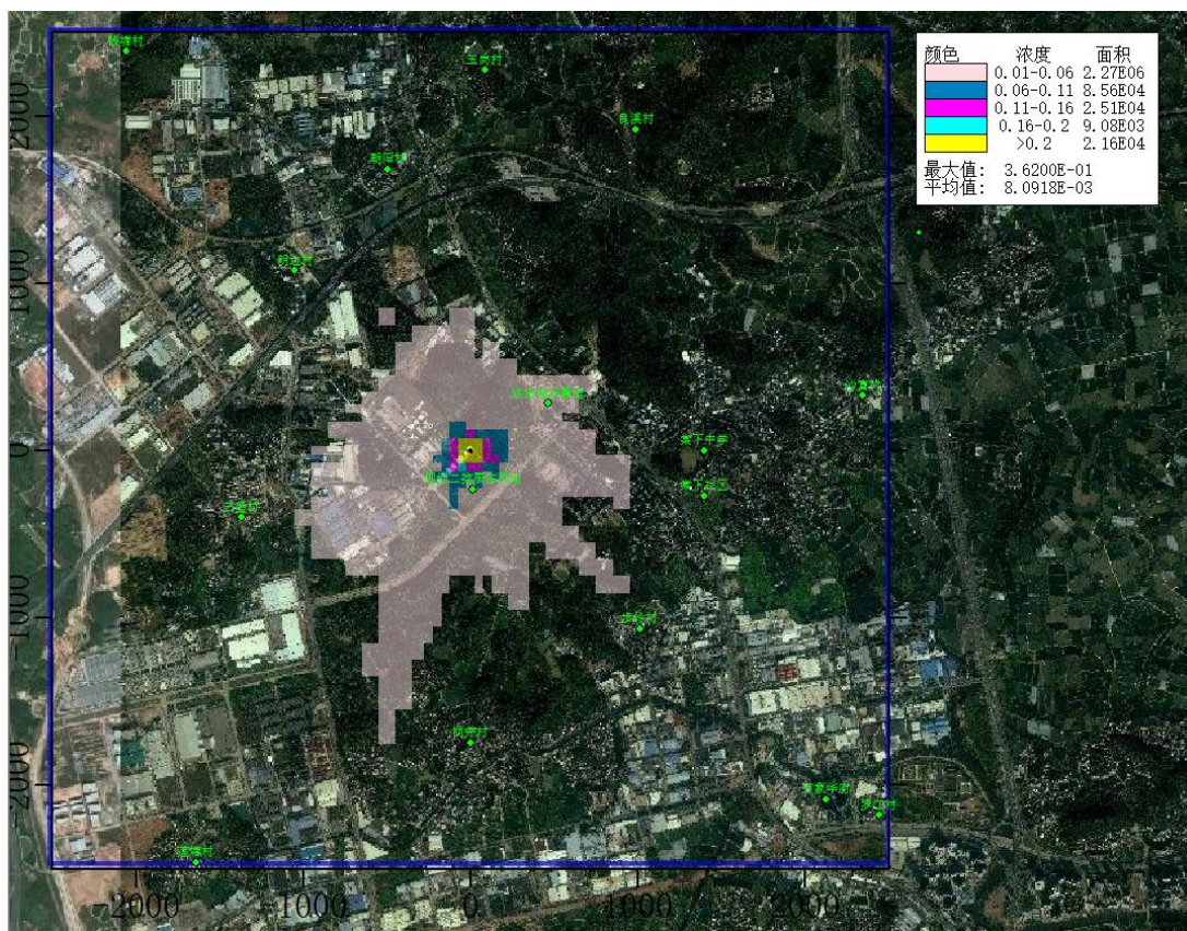
图 5.4.2.2-9 氟化物日平均贡献值等值线图（浓度单位 \mu\text{g}/\text{m}^3 ）
