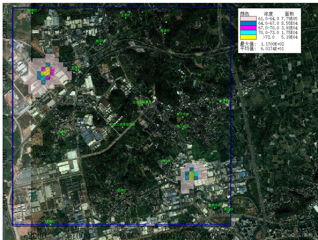
图 5.4.2.2-29 建成后叠加背景值后 TSP 年平均浓度等值线图（浓度单位 \mu\text{g}/\text{m}^3 ）
