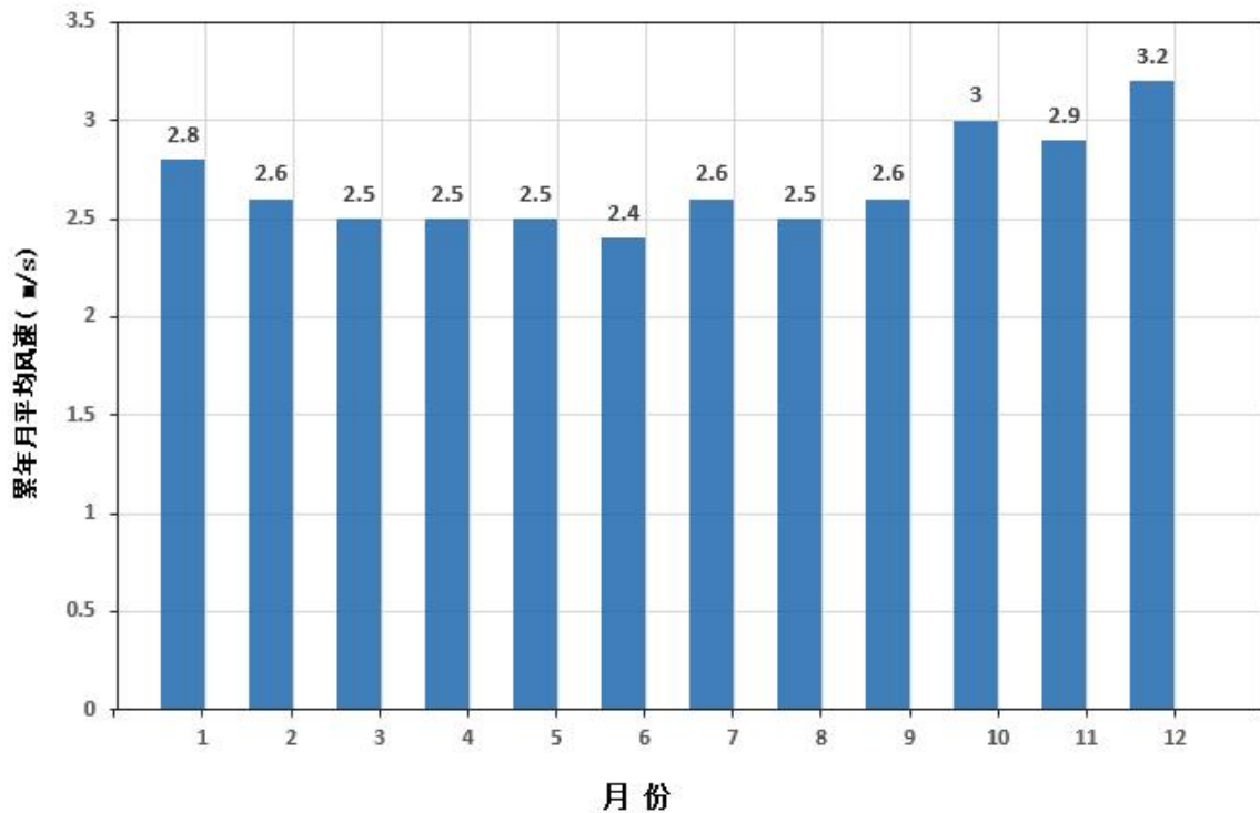
图 4.1.5-1 新会气象站近 20 年 (2004~2023 年) 月平均风速
