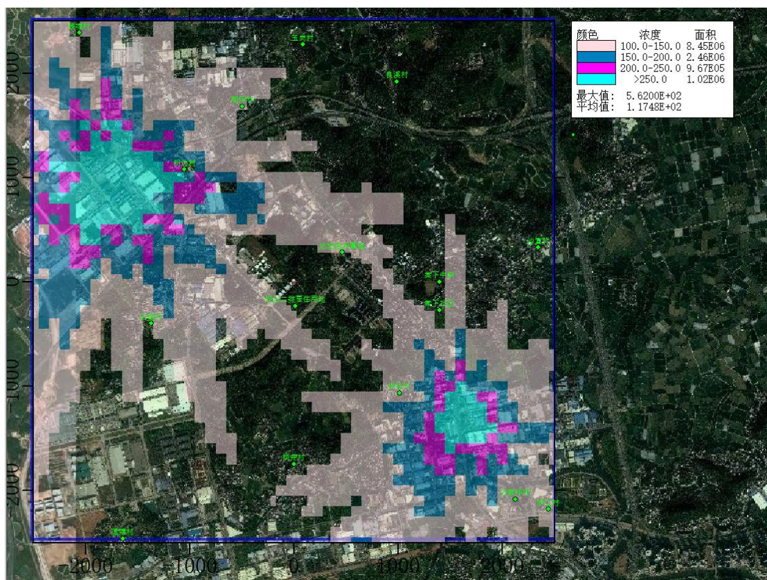
图 5.4.2.2-23 建成后叠加背景值后 TSP 小时浓度等值线图（浓度单位 \mu\text{g}/\text{m}^3 ）
