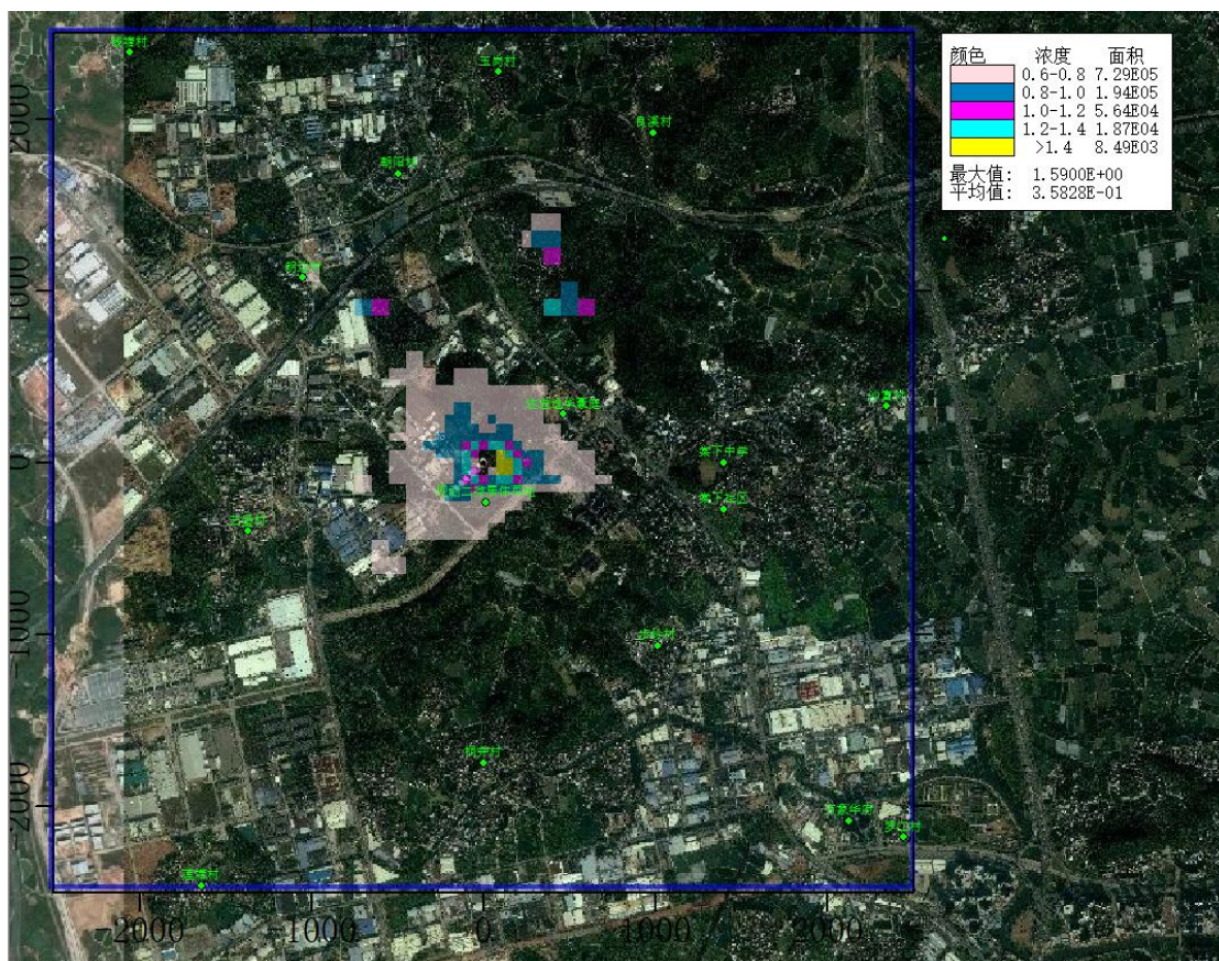
图 5.4.2.2-1 PM 10 小时贡献值等值线图（浓度单位 \mu\text{g}/\text{m}^3 ）
