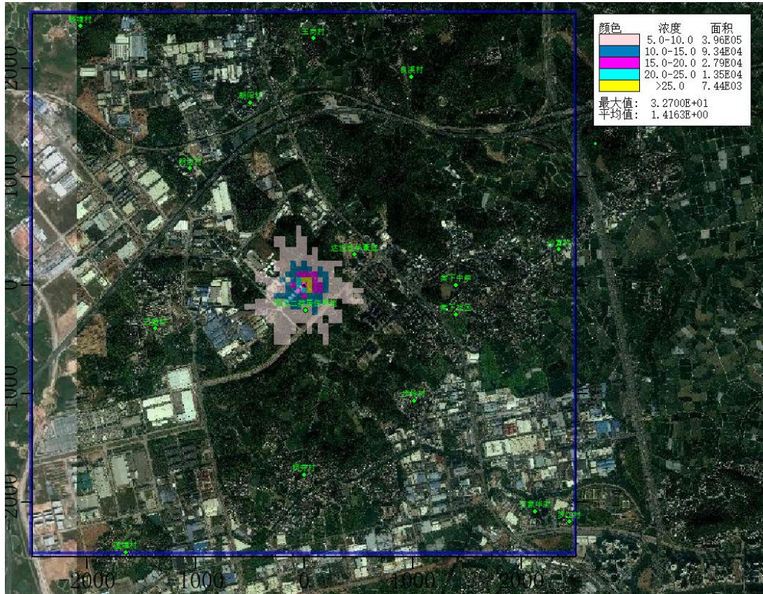
图 5.4.2.2-13 钴及其化合物小时贡献值等值线图（浓度单位 \mu\text{g}/\text{m}^3 ）
