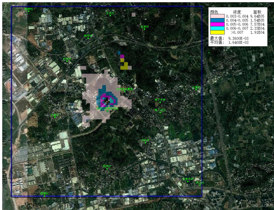
图 5.4.2.2-19 NO 2 年贡献值等值线图（浓度单位 \mu\text{g}/\text{m}^3 ）
