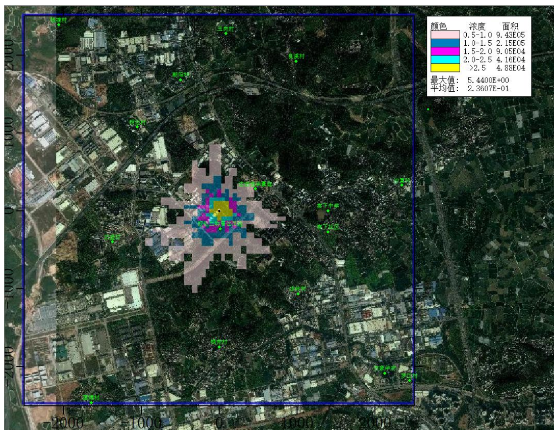
图 5.4.2.2-33 建成后叠加背景值后镍及其化合物小时浓度等值线图（浓度单位 \mu\text{g}/\text{m}^3 ）
