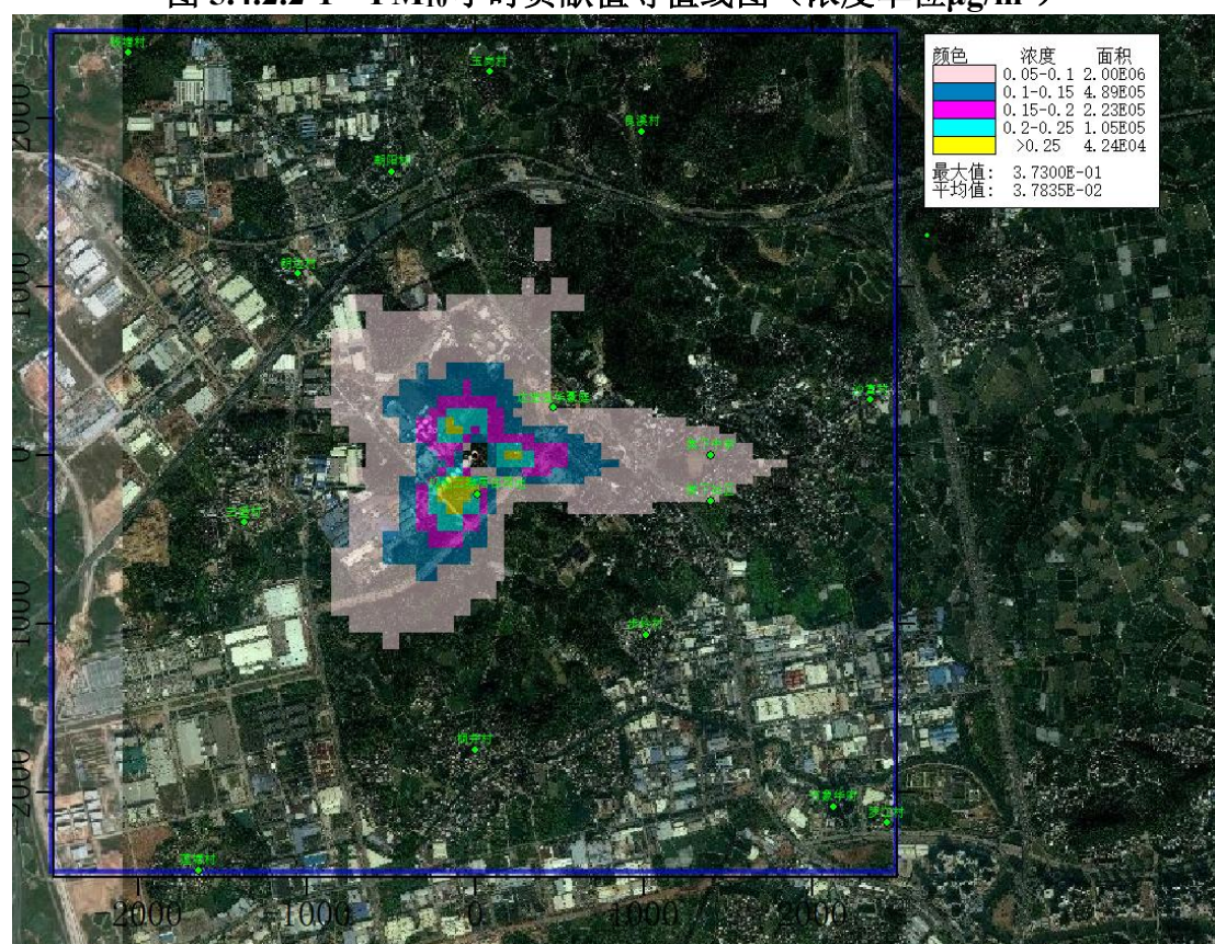
图 5.4.2.2-2 PM 10 日贡献值等值线图（浓度单位 \mu\text{g}/\text{m}^3 ）
