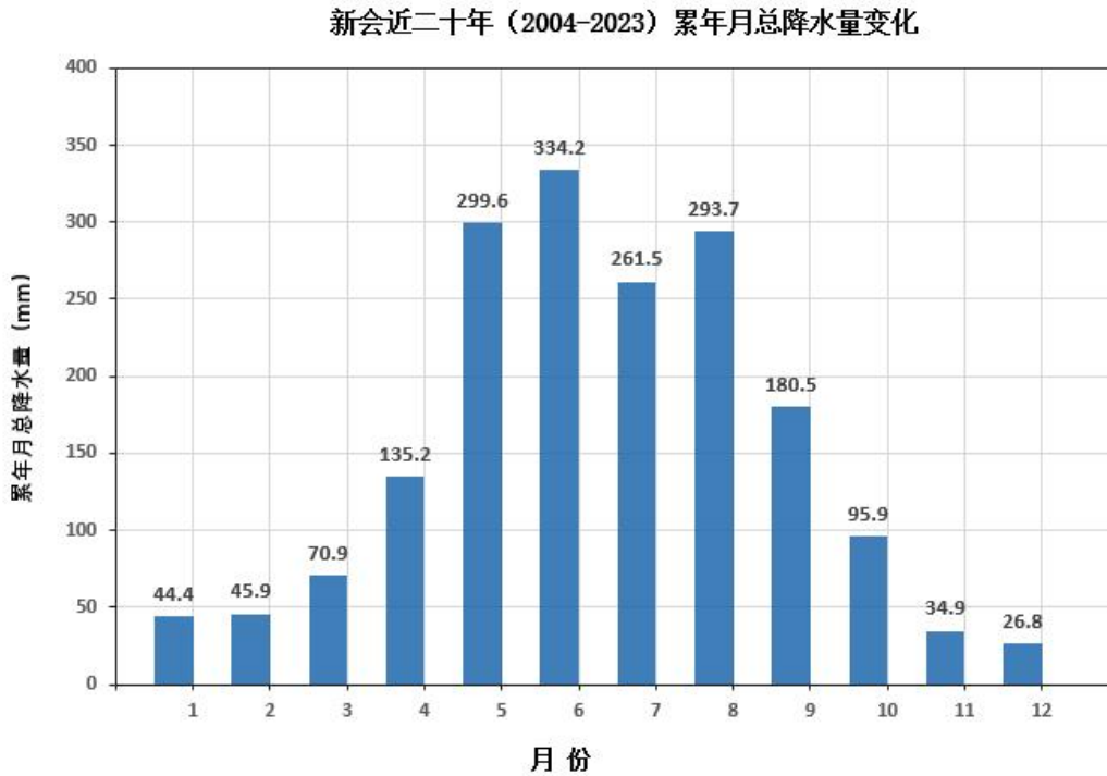
图 4.1.5-6 新会气象站近 20 年(2004~2023 年)月平均降水量
