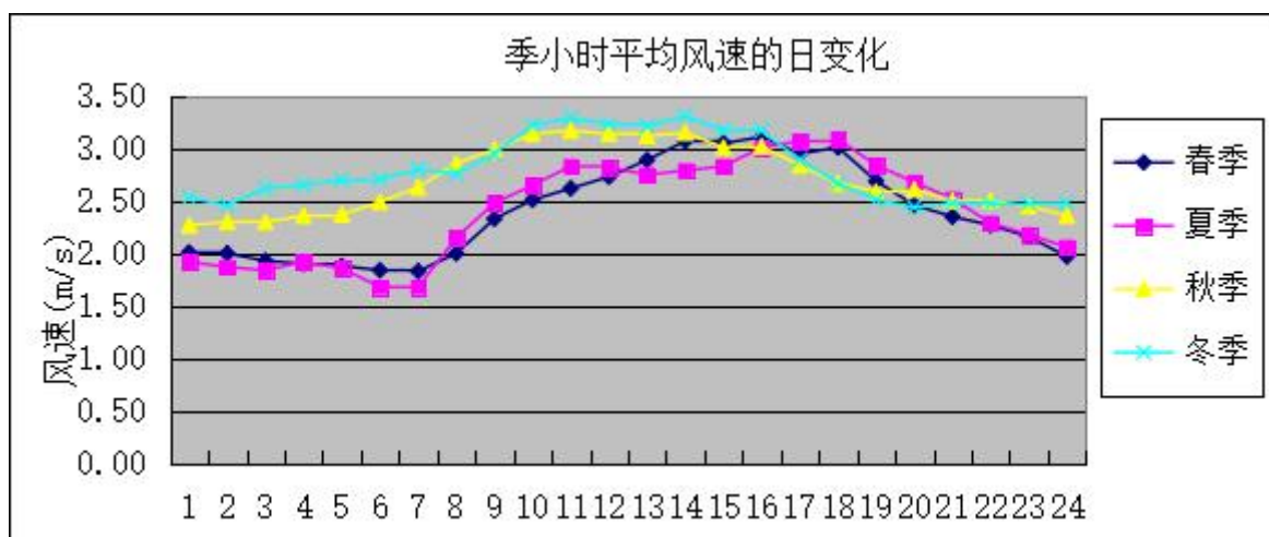
图 4.1.5-14 季小时平均风速的日变化曲线图
