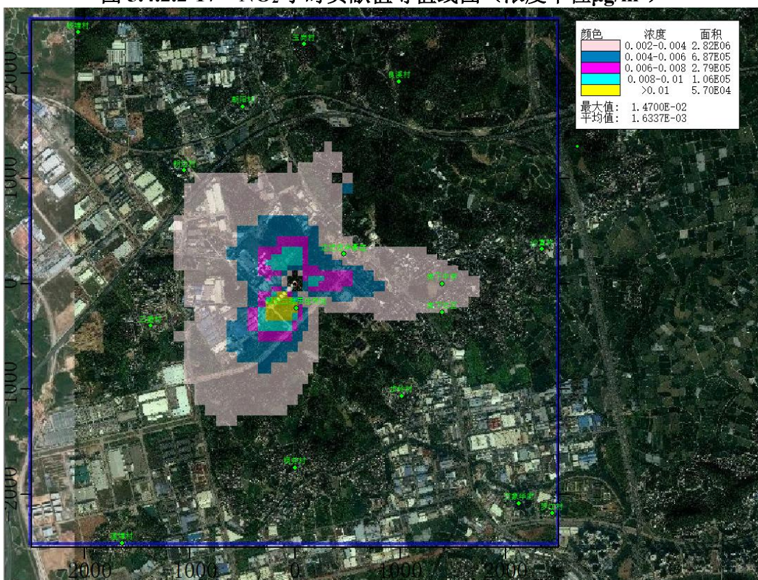
图 5.4.2.2-18 NO 2 日贡献值等值线图（浓度单位 \mu\text{g}/\text{m}^3 ）
