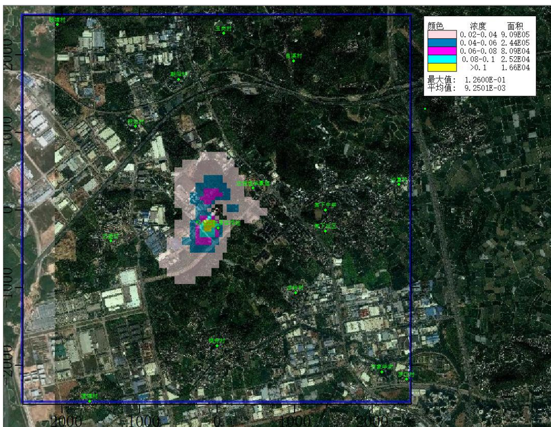
图 5.4.2.2-3 PM 10 年贡献值等值线图（浓度单位 \mu\text{g}/\text{m}^3 ）
