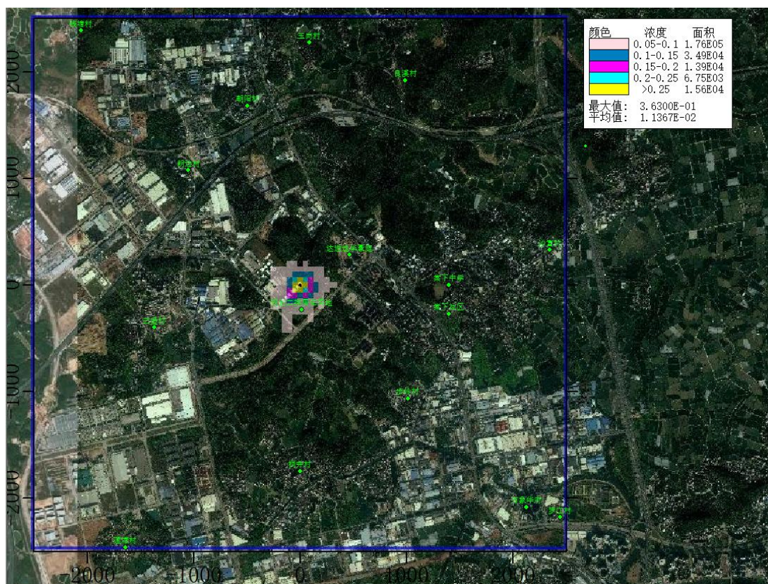
图 5.4.2.2-12 锰及其化合物日平均贡献值等值线图（浓度单位 \mu\text{g}/\text{m}^3 ）
