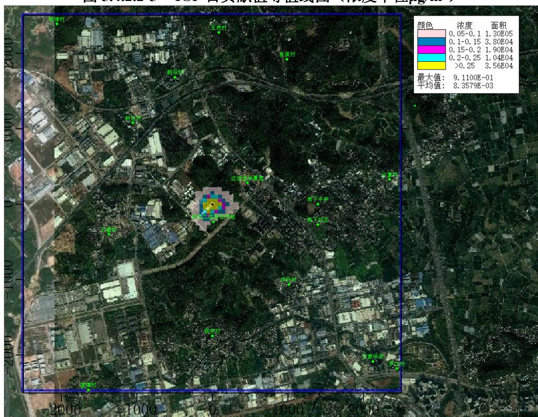
图 5.4.2.2-6 TSP 年贡献值等值线图（浓度单位 \mu\text{g}/\text{m}^3 ）
