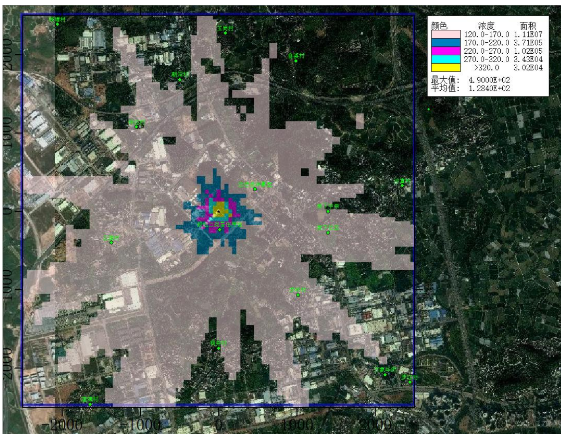
图 5.4.2.2-46 建成后叠加背景值后 TVOC 小浓度等值线图（浓度单位 \mu\text{g}/\text{m}^3 ）
