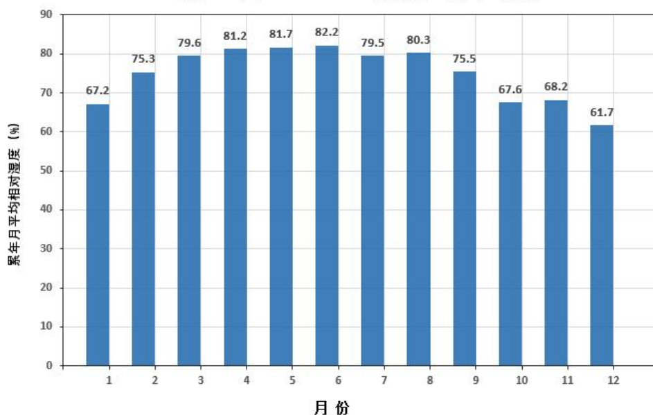
图 4.1.5-10 新会气象站近 20 年(2004~2023 年)月平均相对湿度
