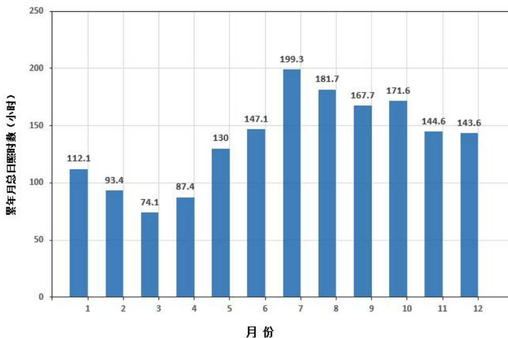
图 4.1.5-8 新会气象站近 20 年(2004~2023 年)月平均日照
