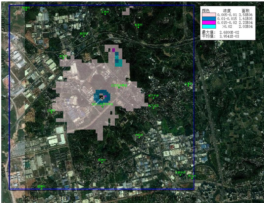
图 5.4.2.2-14 \text{SO}_2 小时贡献值等值线图（浓度单位 \mu\text{g}/\text{m}^3 ）
