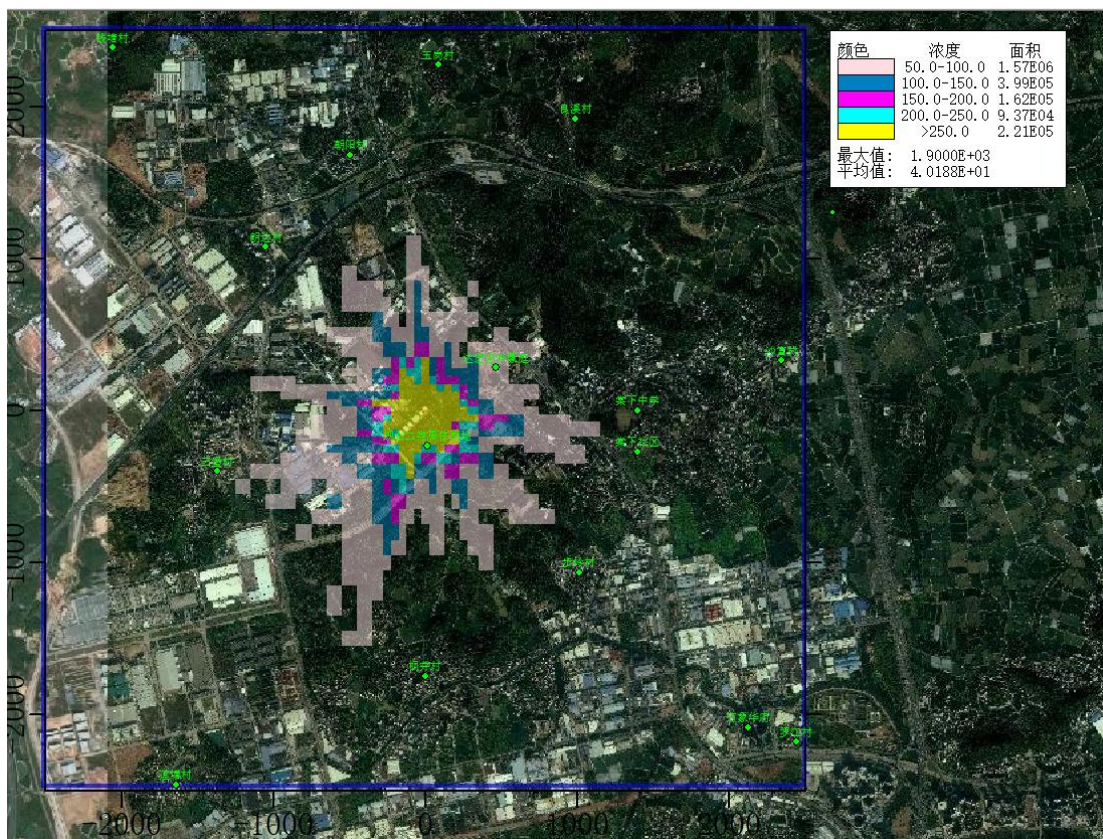
图 5.4.2.2-52 非正常工况下锰及其化合物小时贡献值等值线图（浓度单位 \mu\text{g}/\text{m}^3 ）
