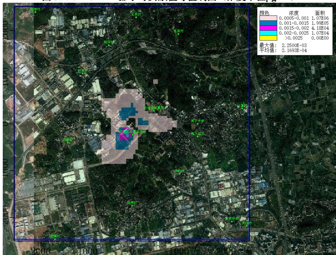
图 5.4.2.2-21 PM 2.5 日贡献值等值线图（浓度单位 \mu\text{g}/\text{m}^3 ）
