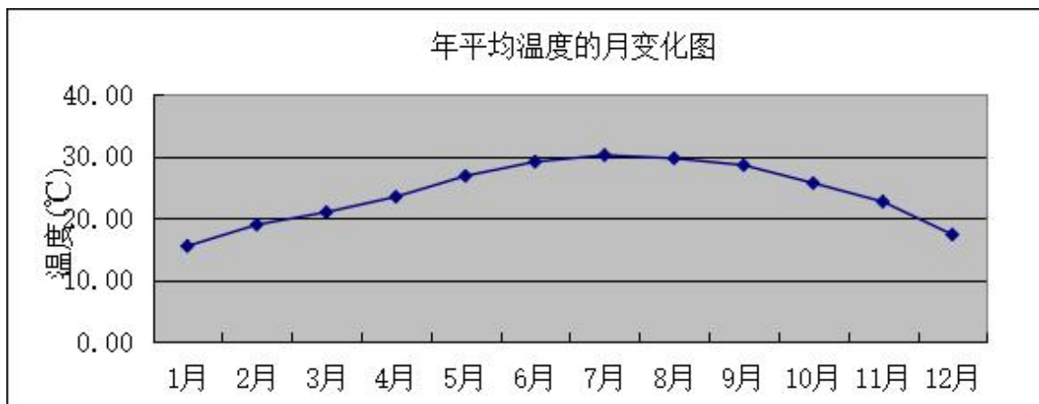
图 4.1.5-12 年平均温度月变化曲线图
