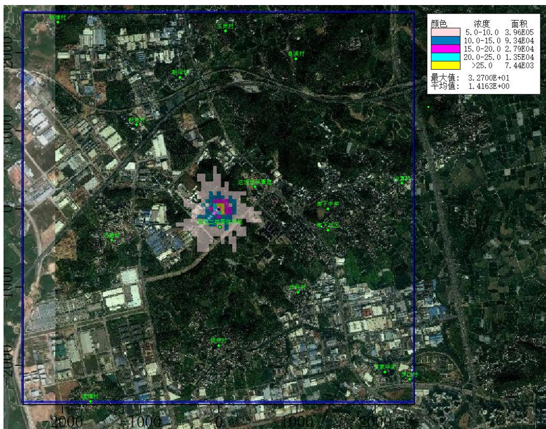
图 5.4.2.2-36 建成后叠加背景值后钴及其化合物小时浓度等值线图(浓度单位 \mu\text{g}/\text{m}^3 )
