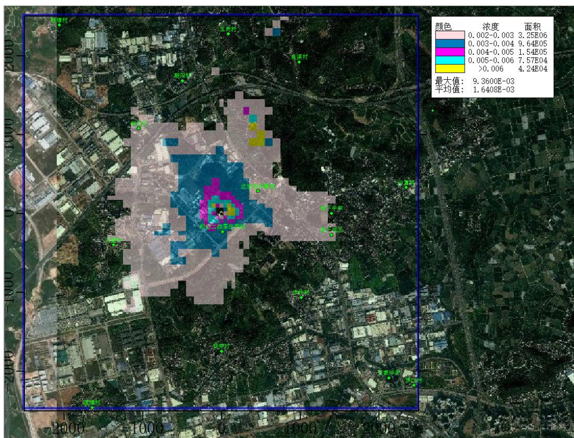
图 5.4.2.2-43 建成后叠加背景值后 PM 2.5 小时浓度等值线图（浓度单位 \mu\text{g}/\text{m}^3 ）
