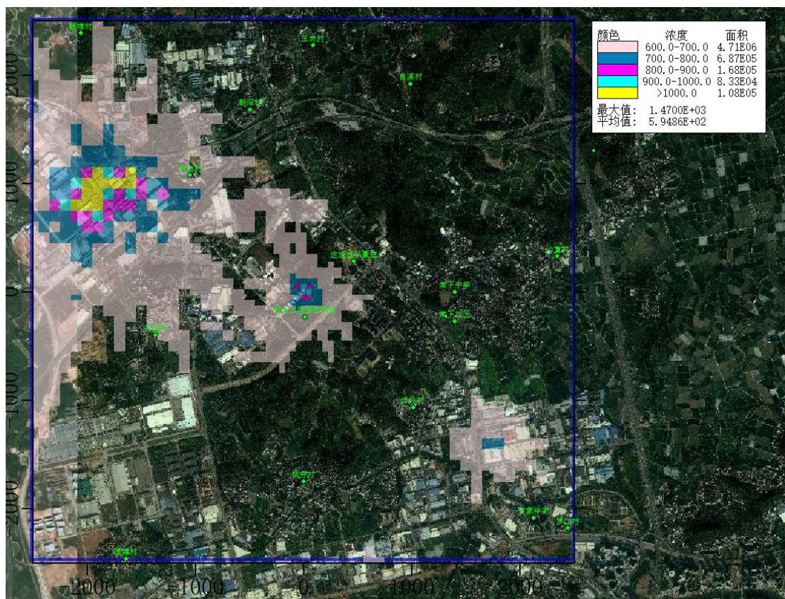
图 5.4.2.2-30 建成后叠加背景值后非甲烷总烃小时浓度等值线图（浓度单位 \mu\text{g}/\text{m}^3 ）
