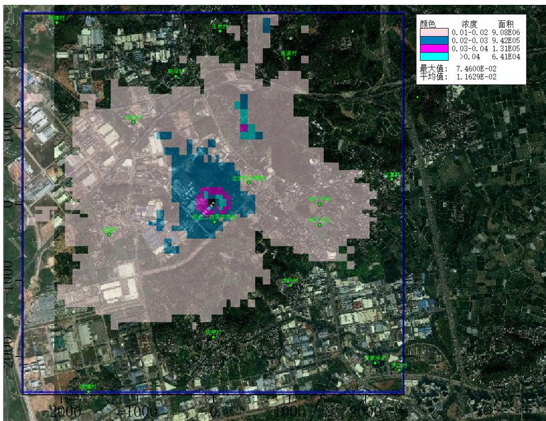
图 5.4.2.2-40 建成后叠加背景值后 NO 2 小时浓度等值线图（浓度单位 \mu\text{g}/\text{m}^3 ）
