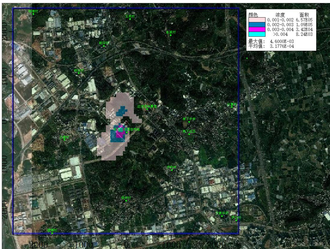
图 5.4.2.2-42 建成后叠加背景值后 NO 2 年平均浓度等值线图（浓度单位 \mu\text{g}/\text{m}^3 ）
