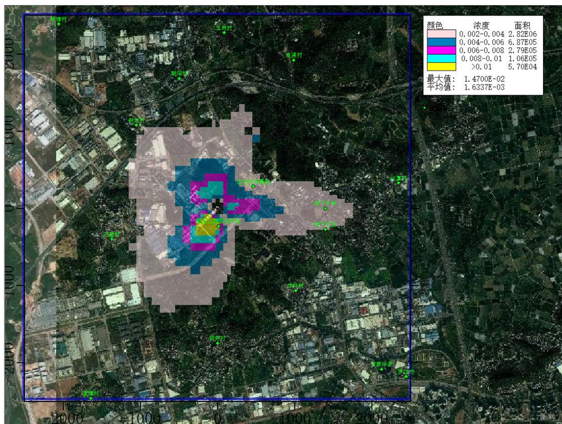
图 5.4.2.2-41 建成后叠加背景值后 NO 2 日平均浓度等值线图（浓度单位 \mu\text{g}/\text{m}^3 ）
