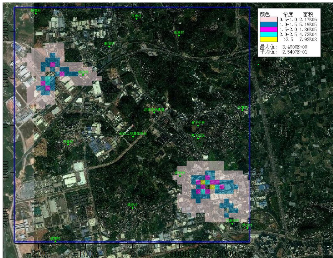
图 5.4.2.2-26 建成后叠加背景值后 PM 10 日平均浓度等值线图（浓度单位 \mu\text{g}/\text{m}^3 ）
