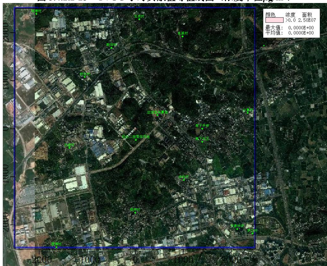
图 5.4.2.2-24 二噁英年贡献值等值线图（浓度单位 \mu\text{g}/\text{m}^3 ）
