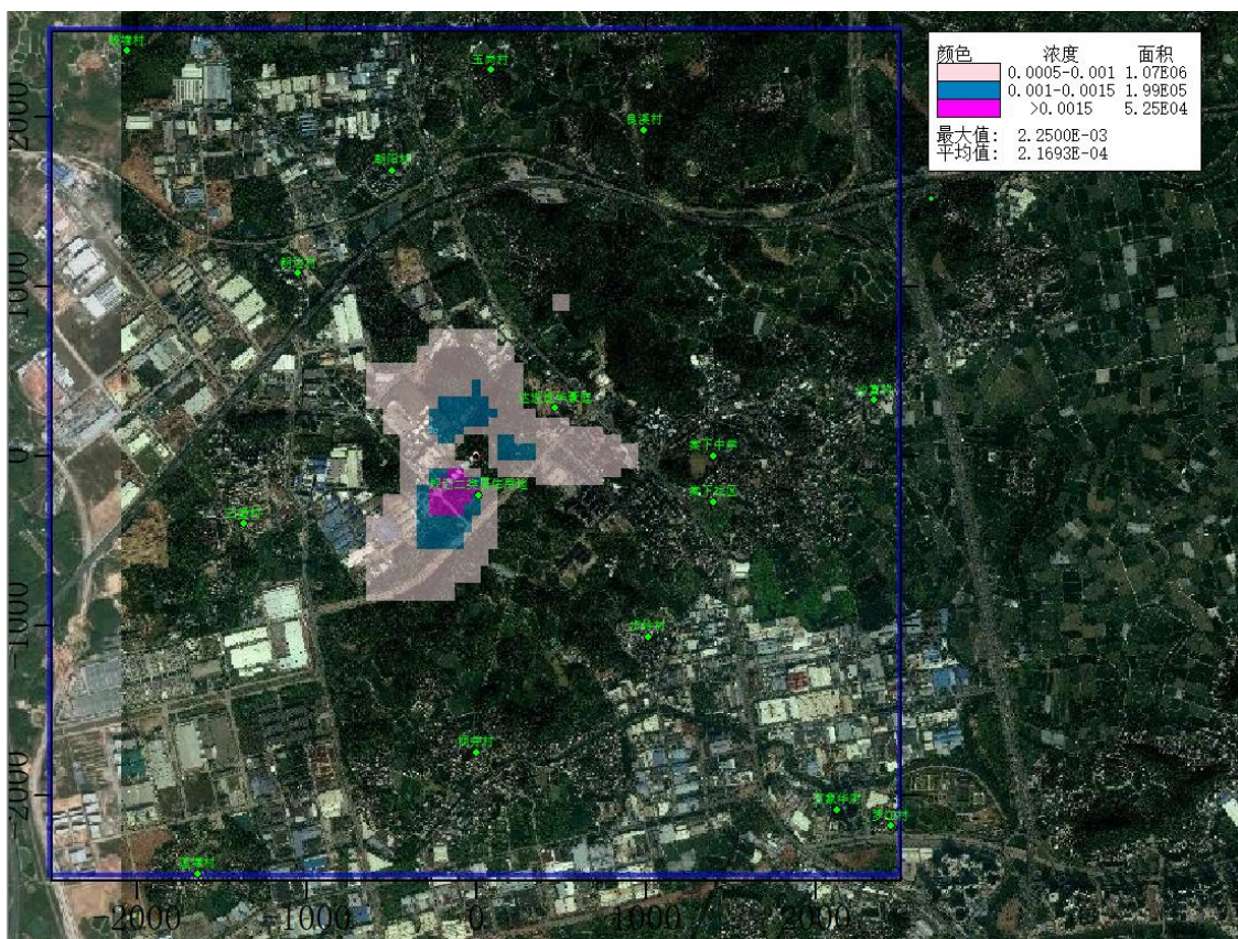
图 5.4.2.2-44 建成后叠加背景值后 PM 2.5 日平均浓度等值线图（浓度单位 \mu\text{g}/\text{m}^3 ）
