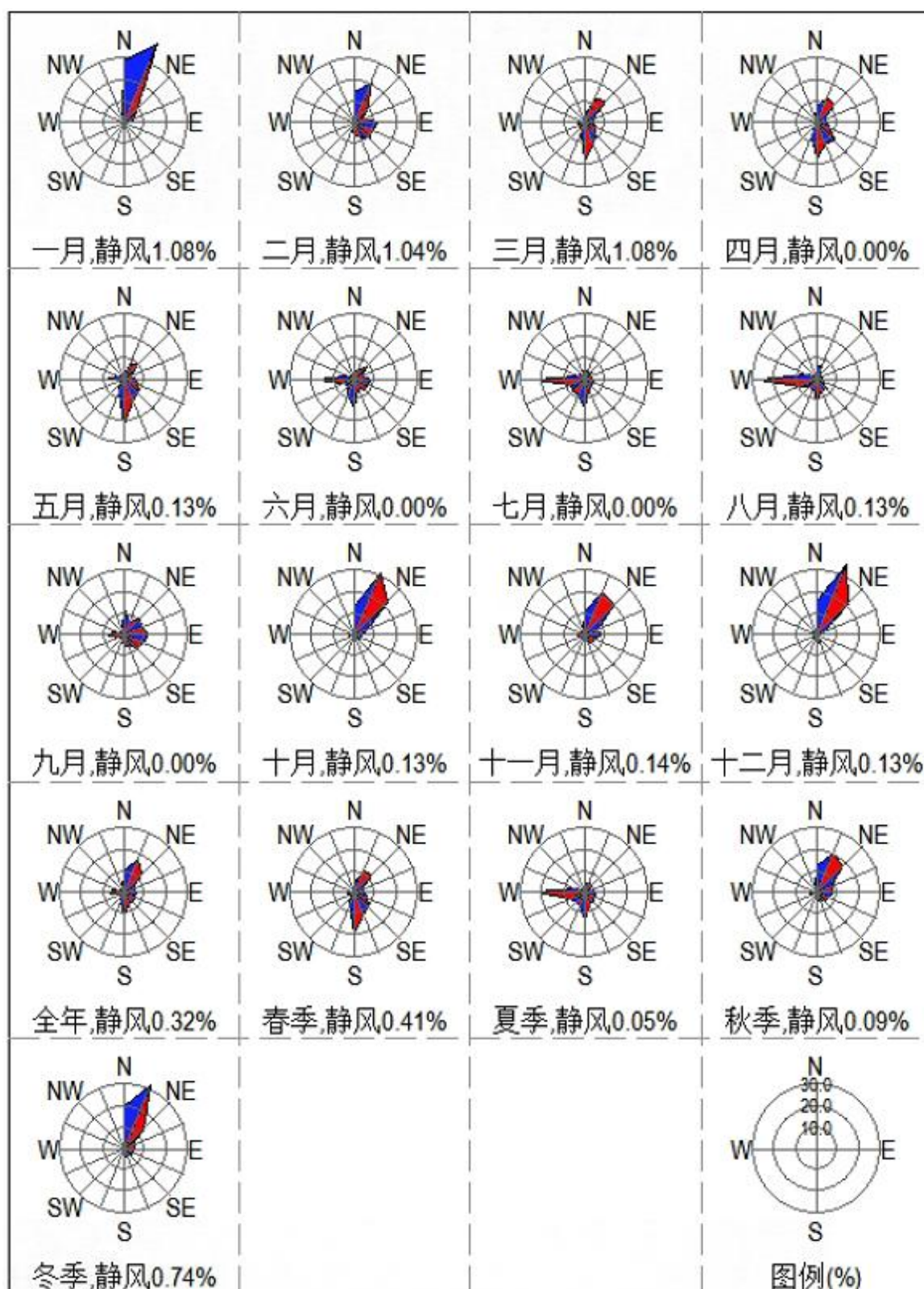
图 4.1.5-15 新会气象 2023 年风频玫瑰图
