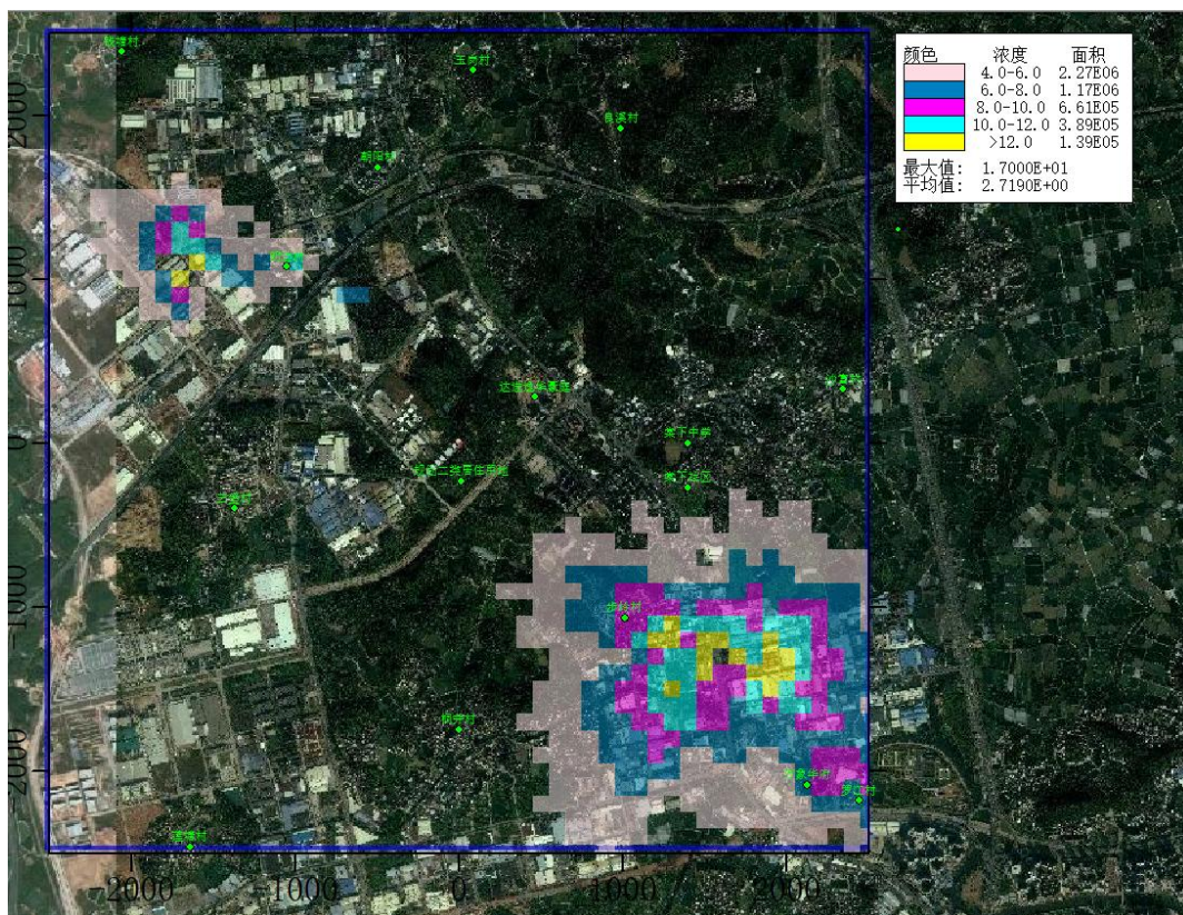
图 5.4.2.2-25 建成后叠加背景值后 PM 10 小时平均浓度等值线图（浓度单位 \mu\text{g}/\text{m}^3 ）
