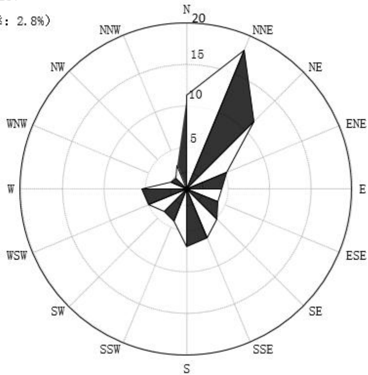
图 4.1.5-2 新会气象站近 20 年（2004~2023 年）年平均风向风频玫瑰图
