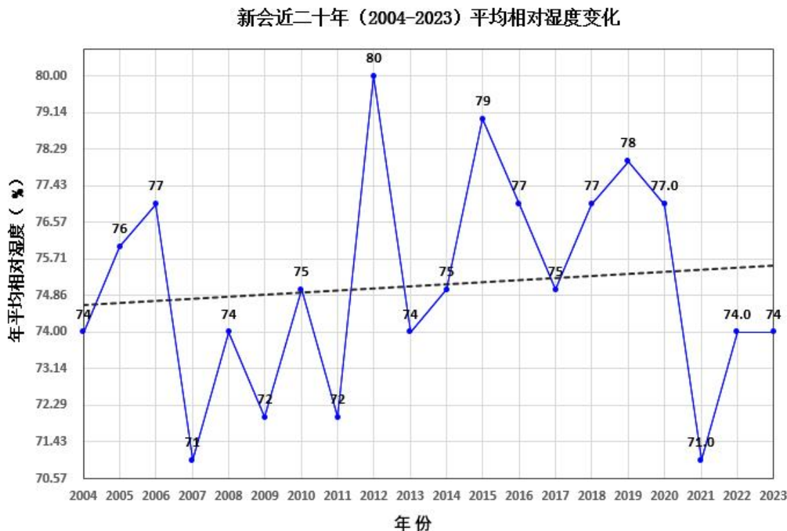
图 4.1.5-11 新会气象站近 20 年(2004~2023 年)年平均相对湿度
