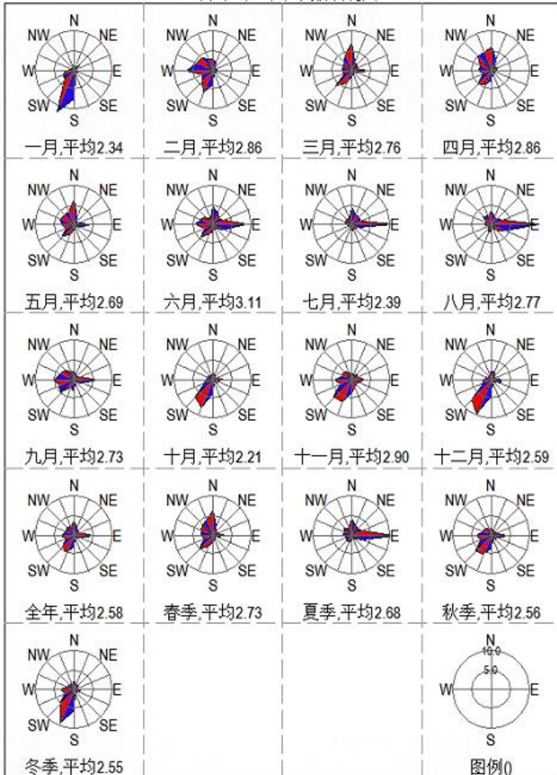
图4.1.5-16 2023年各风向污染系数玫瑰图
