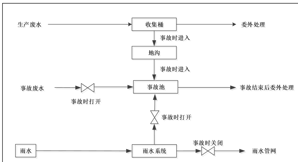
图 6.4.3-1 防止事故水进入外环境的控制、封堵系统图
