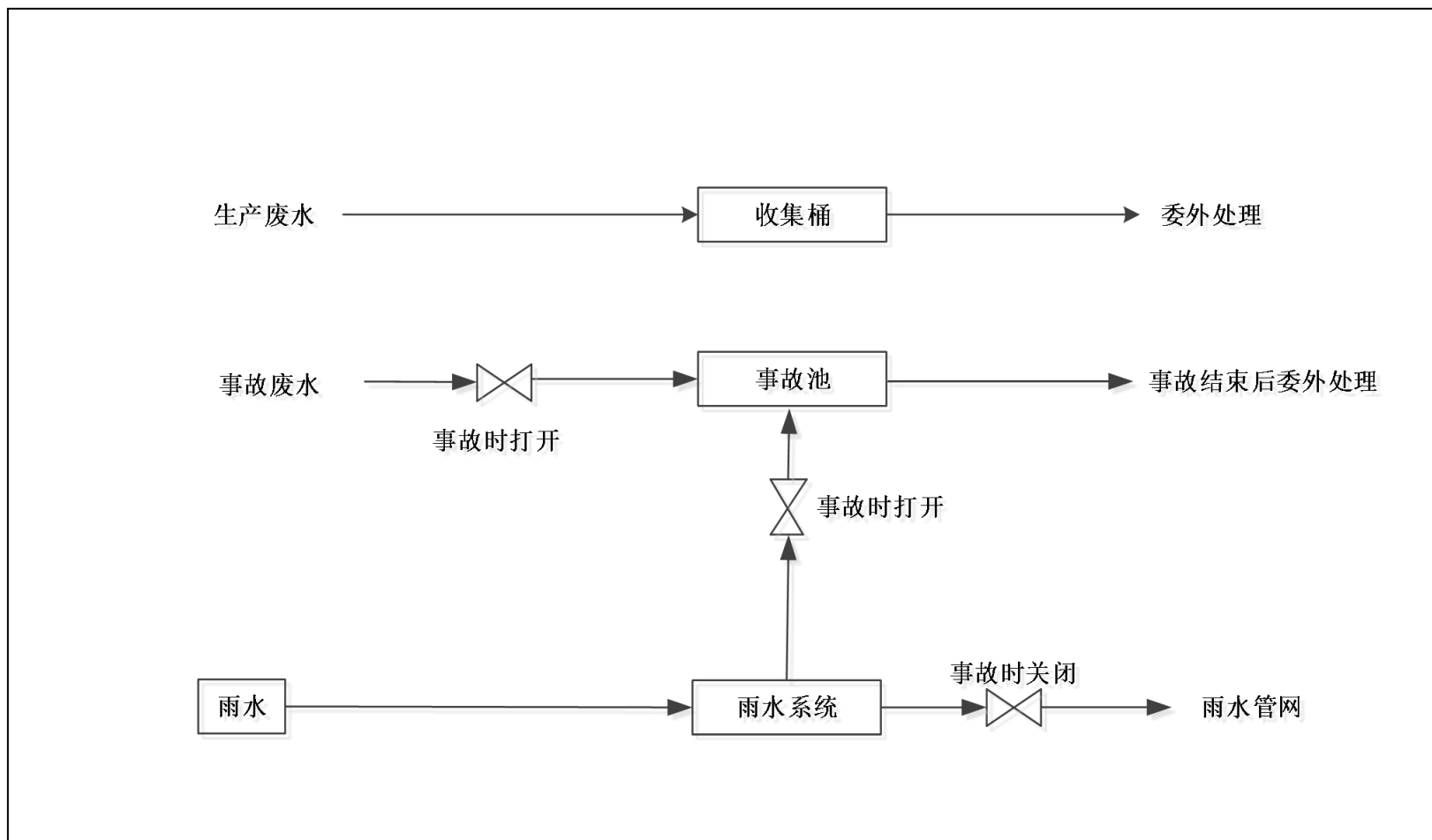
图 5.7.7-2 防止事故水进入外环境的控制、封堵系统图
