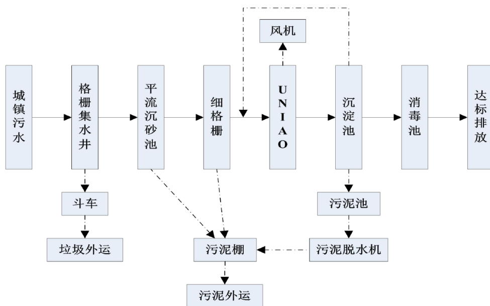
图7-28 共和污水处理厂污水处理工艺流程图
