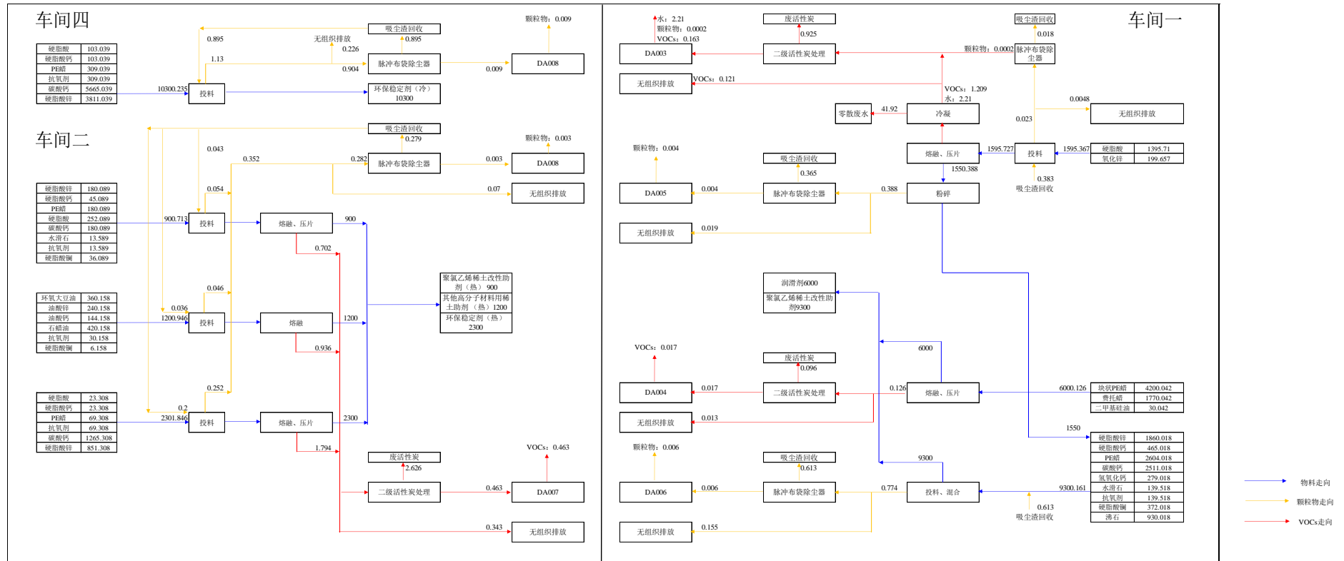
图4-18 物料平衡图
