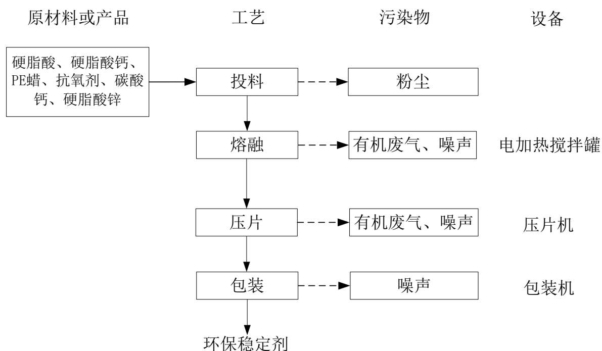
图4-16 环保稳定剂生产工艺
