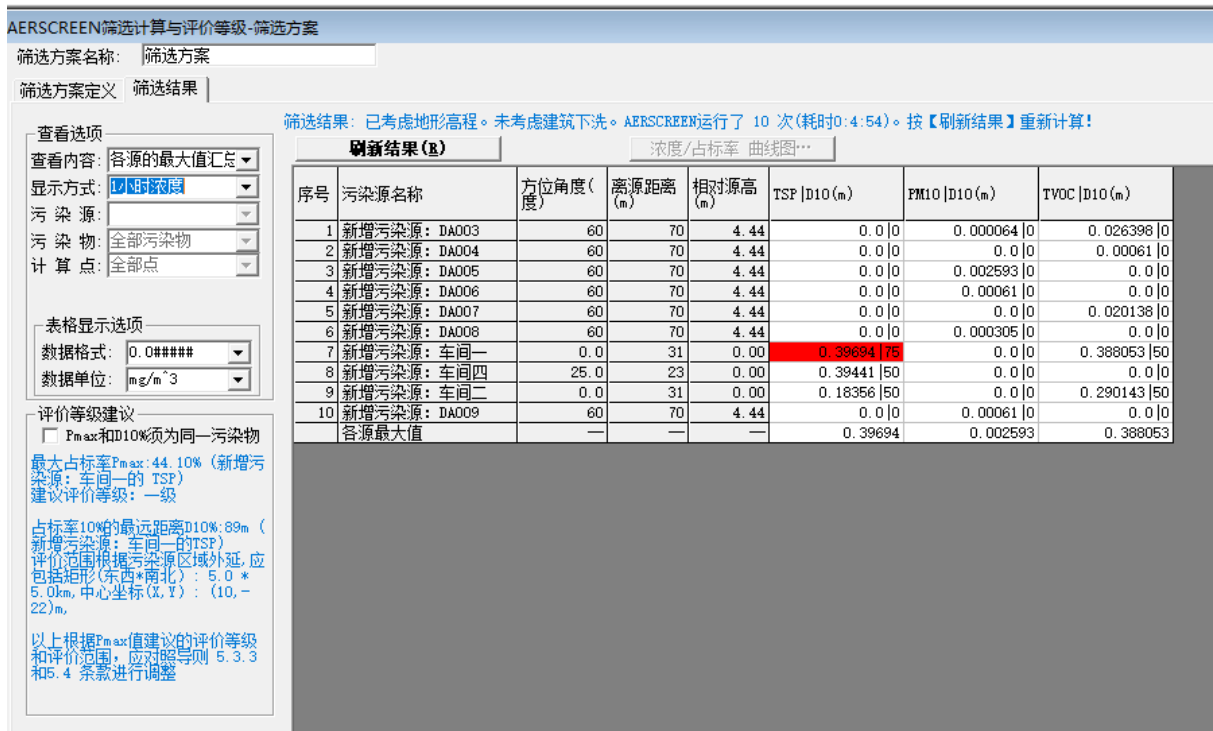
图2-6 估算模式 AERSCREEN 点源、面源截图
