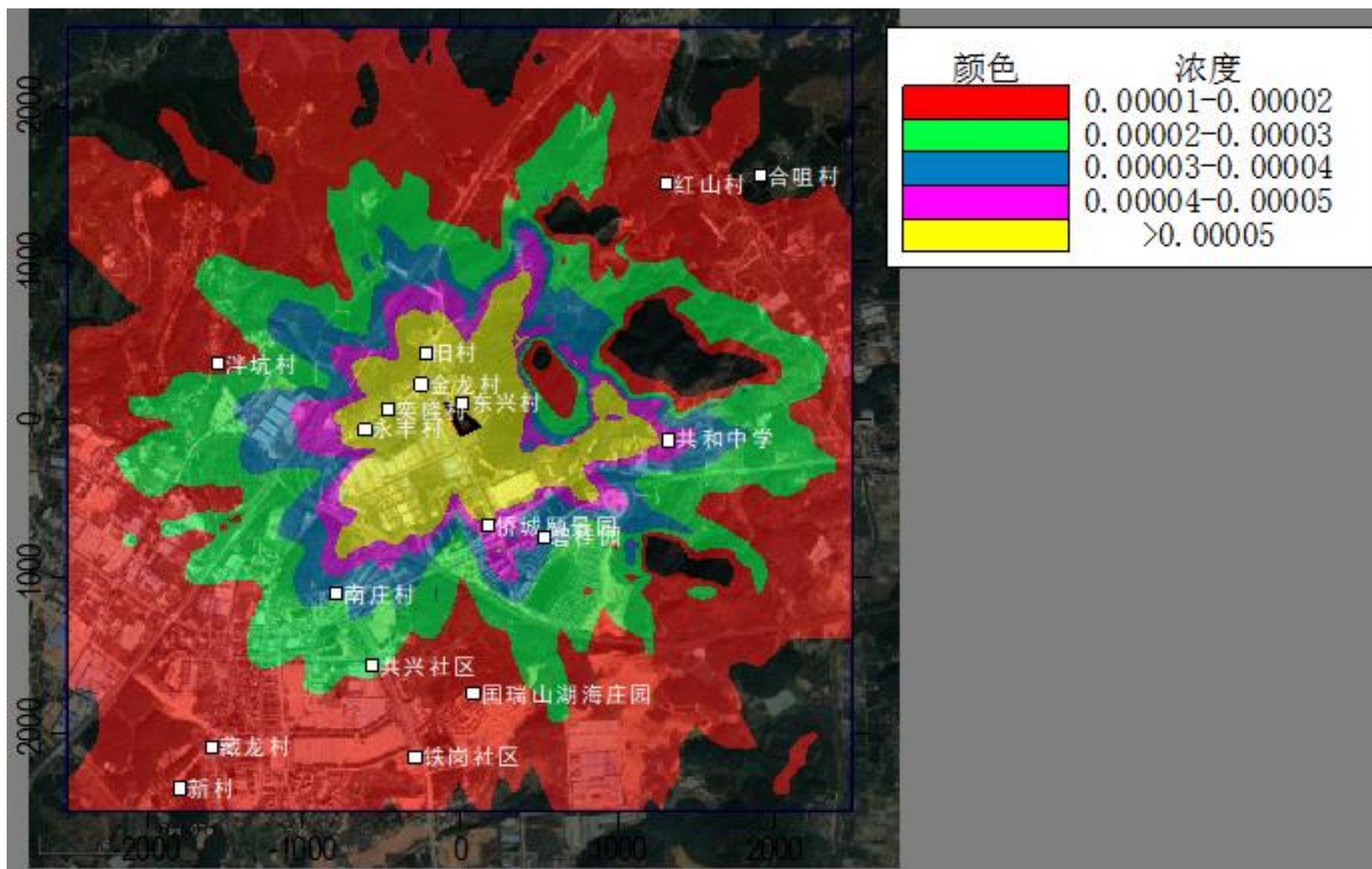
图7-17 新增 PM 2.5 日平均质量浓度分布图
