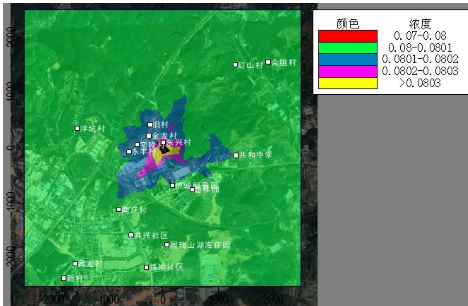
图7-15 叠加后 PM 10 日平均质量浓度分布图
