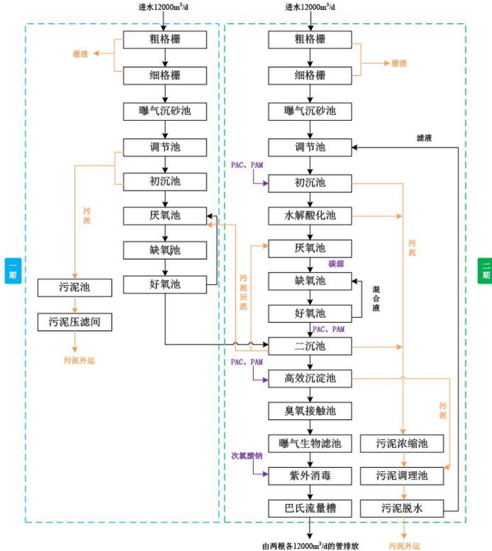
图5.3-2污水处理厂水处理工艺流程图
