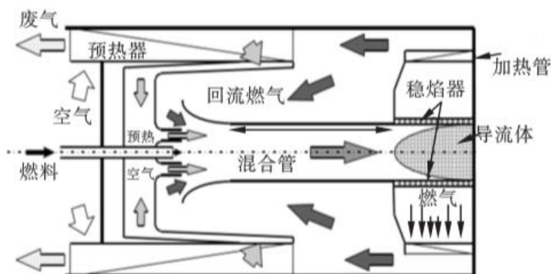
图6.1-1同类型低氮燃烧器示意图
