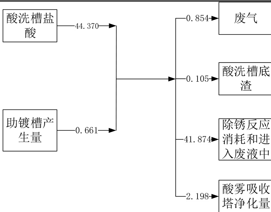
图3.3-2 本工程氯平衡图
