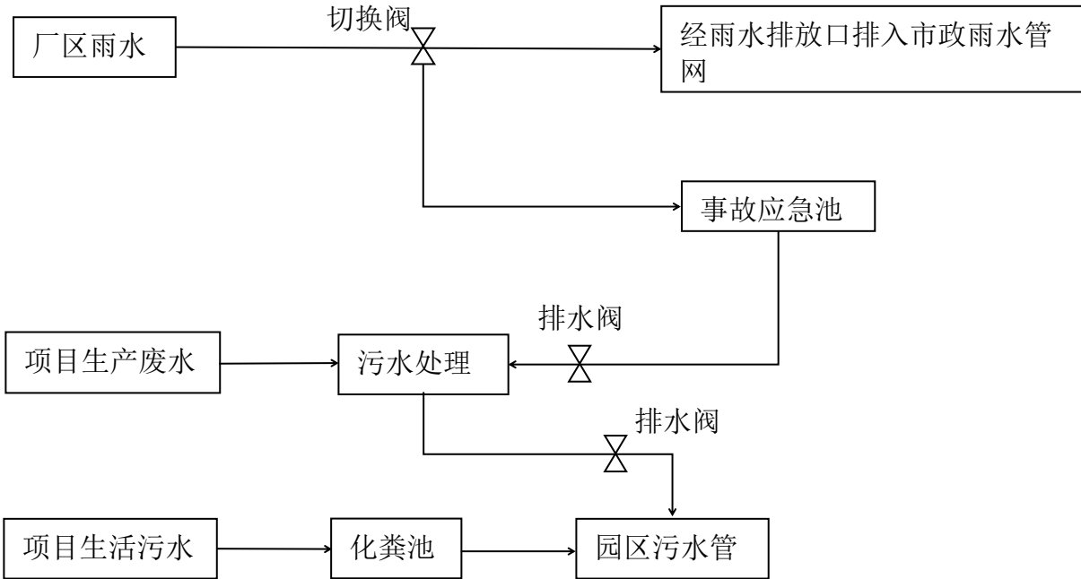
图5.9-4 防止事故水进入外环境的控制、封堵措施图
