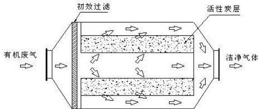
图 6.1-1 活性炭固定吸附装置示意图
