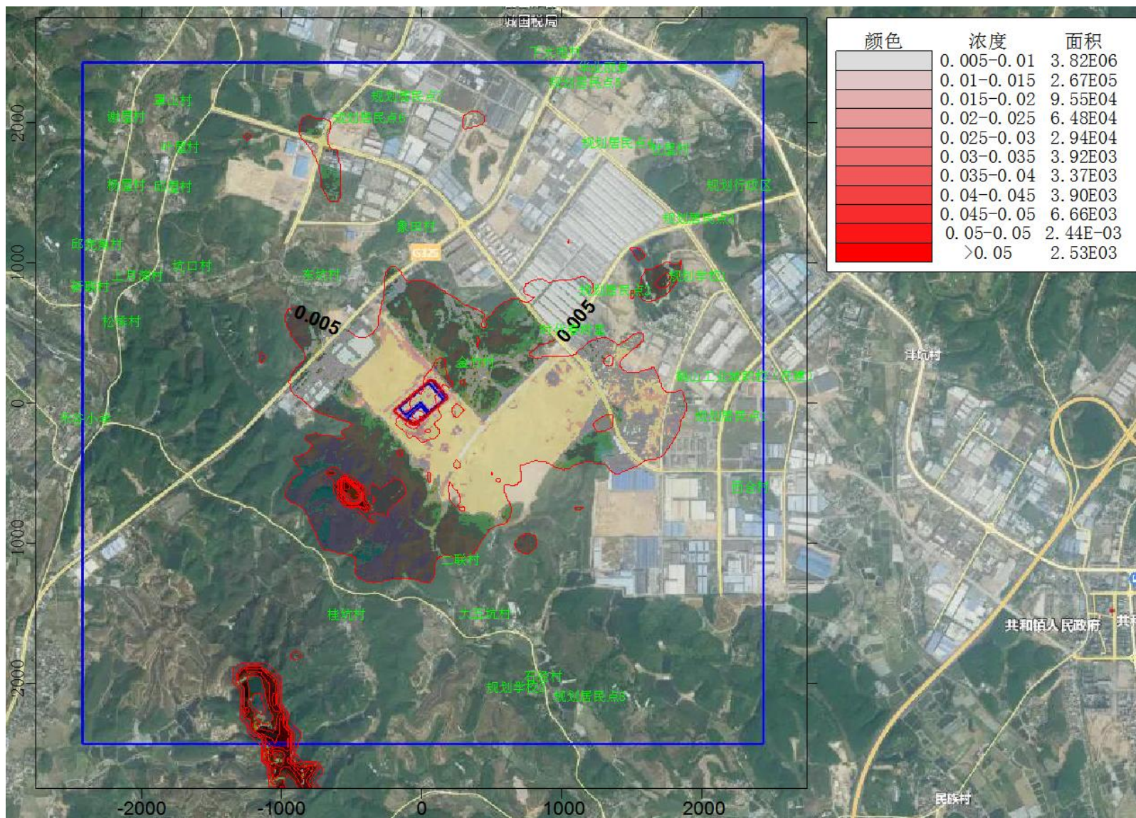
图 5.2-49 非正常排放 PM 2.5 最大小时质量浓度分布图
