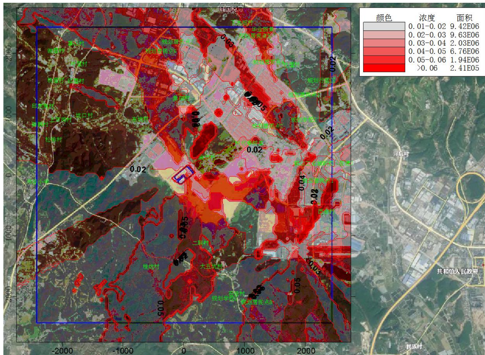
图 5.2-38 NO x 叠加区域在建拟建污染源和现状背景浓度保证率日平均质量浓度分布图
