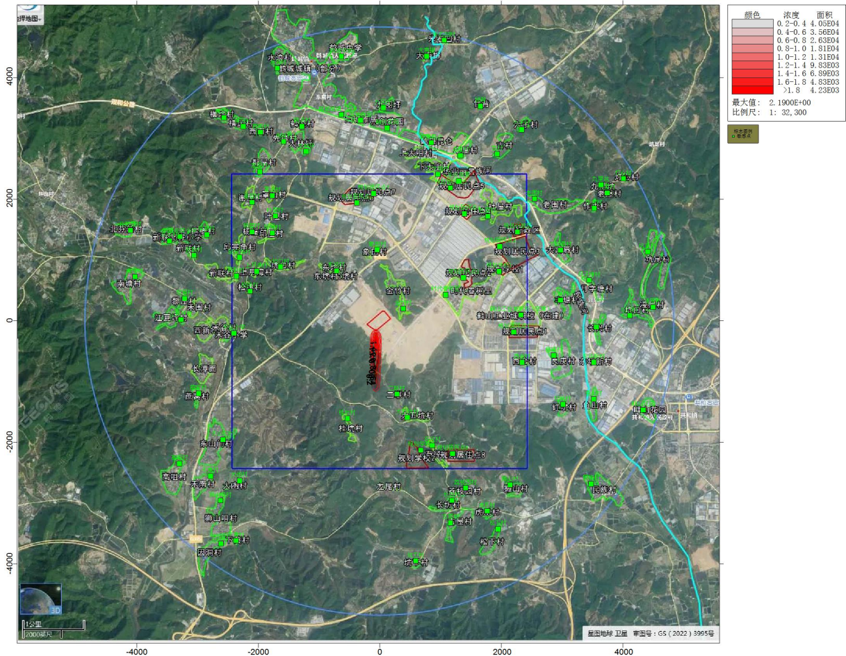
图5.9-3 不利气象条件下废气事故排放的氯化氢等值线图
