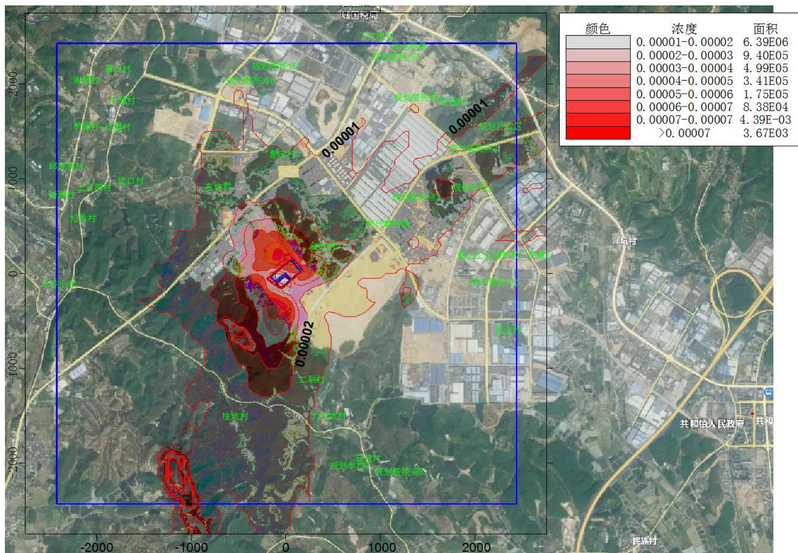
图 5.2-28 PM 2.5 新增污染源最日平均贡献浓度分布图
