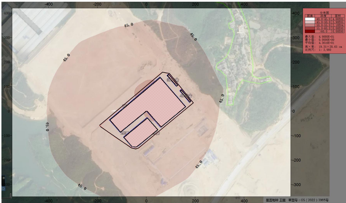
图 5.5-2 昼间噪声贡献值等声级线图
