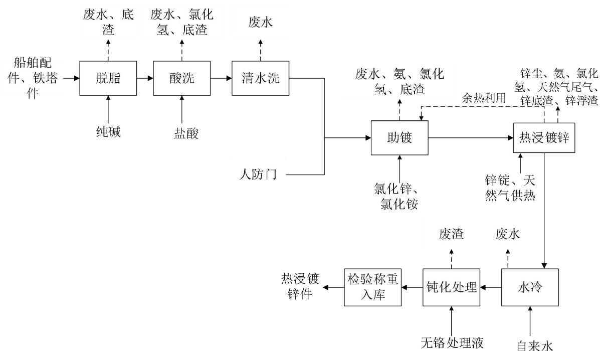
图 3.2-2 热浸镀锌工艺流程图
