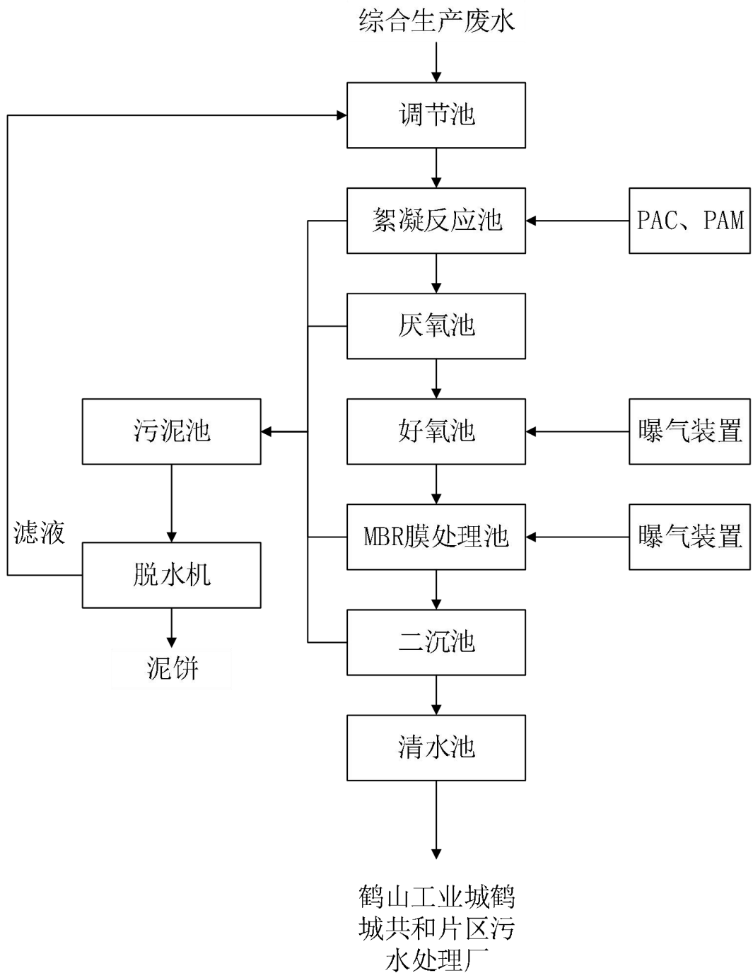
图 6.1-2 生产废水处理工艺流程图
