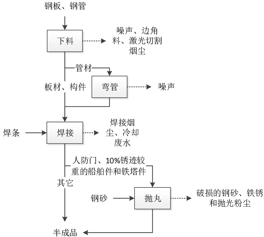
图3.2-1 机加工工艺流程及产污环节图
