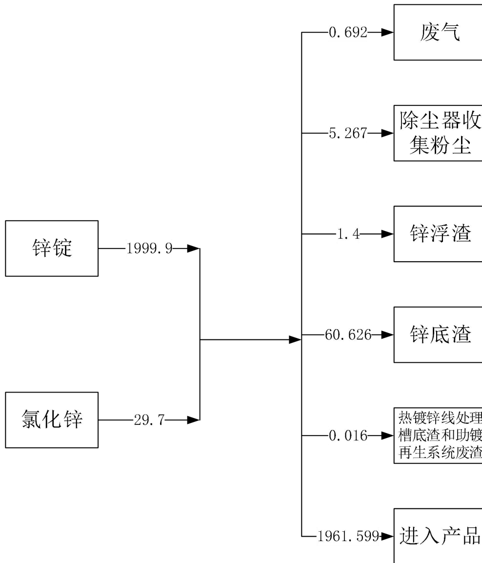
图3.3-1 本工程锌元素平衡图
