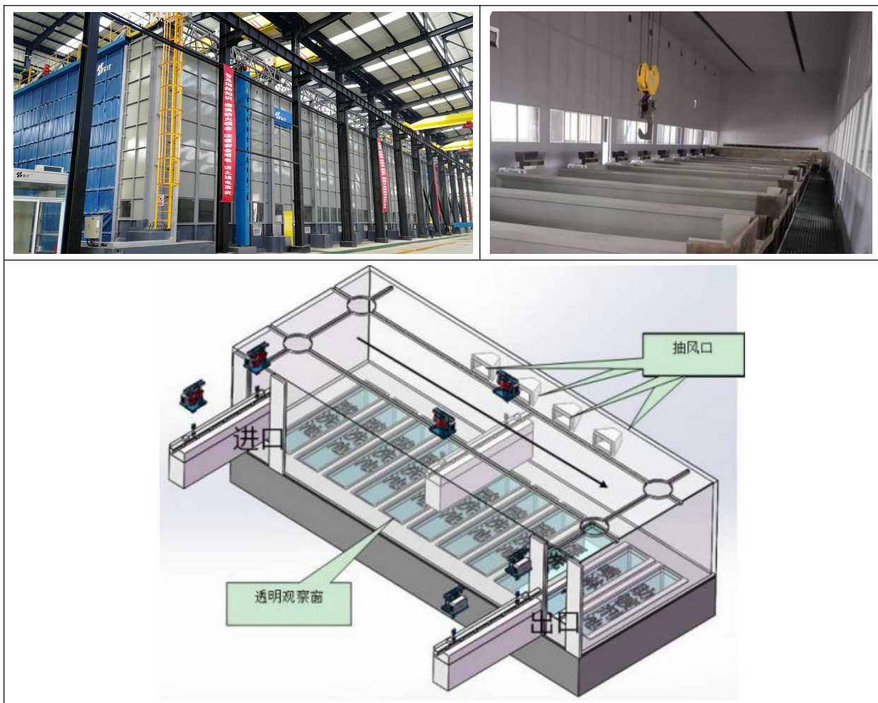
图3.5-1同类型全封闭热镀锌酸洗线示意图
