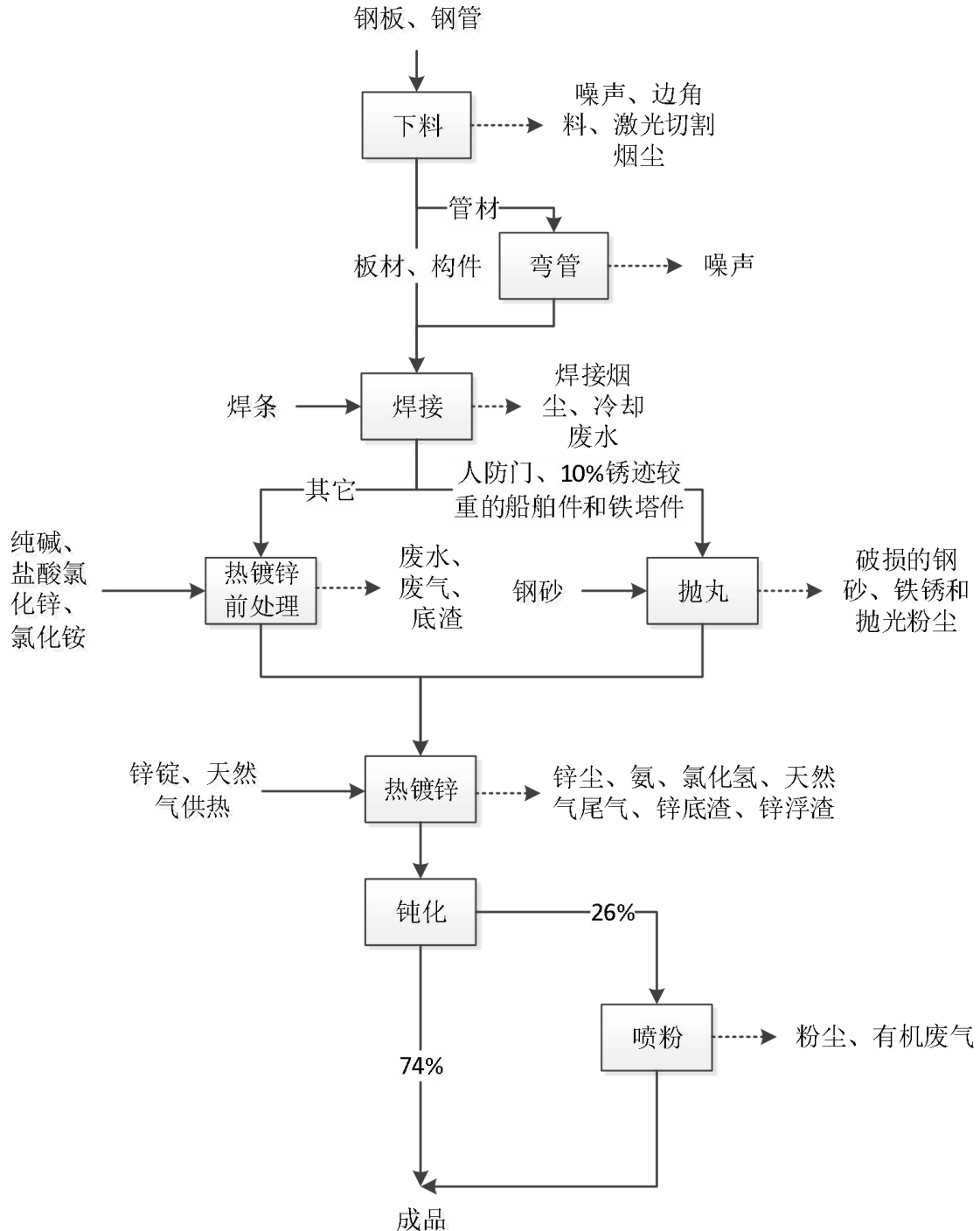
图3.2-4总工艺流程图
