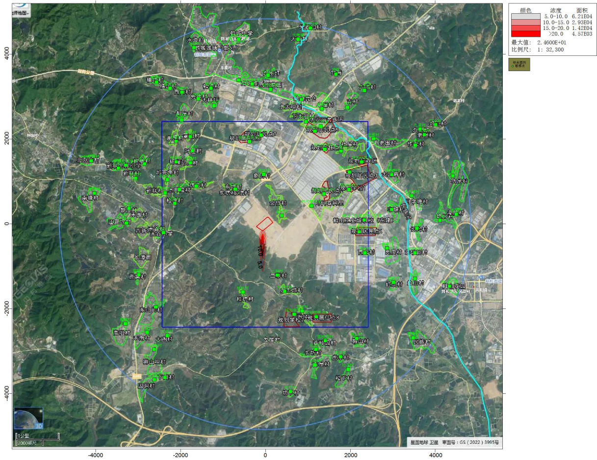
图5.9-2 不利气象条件下液池挥发的氯化氢等值线图
