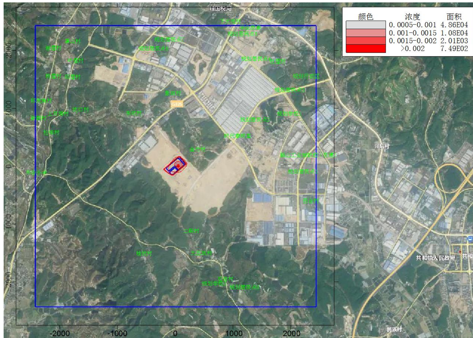
图5.2-25 NO 2 新增污染源最大年平均质量浓度分布图
