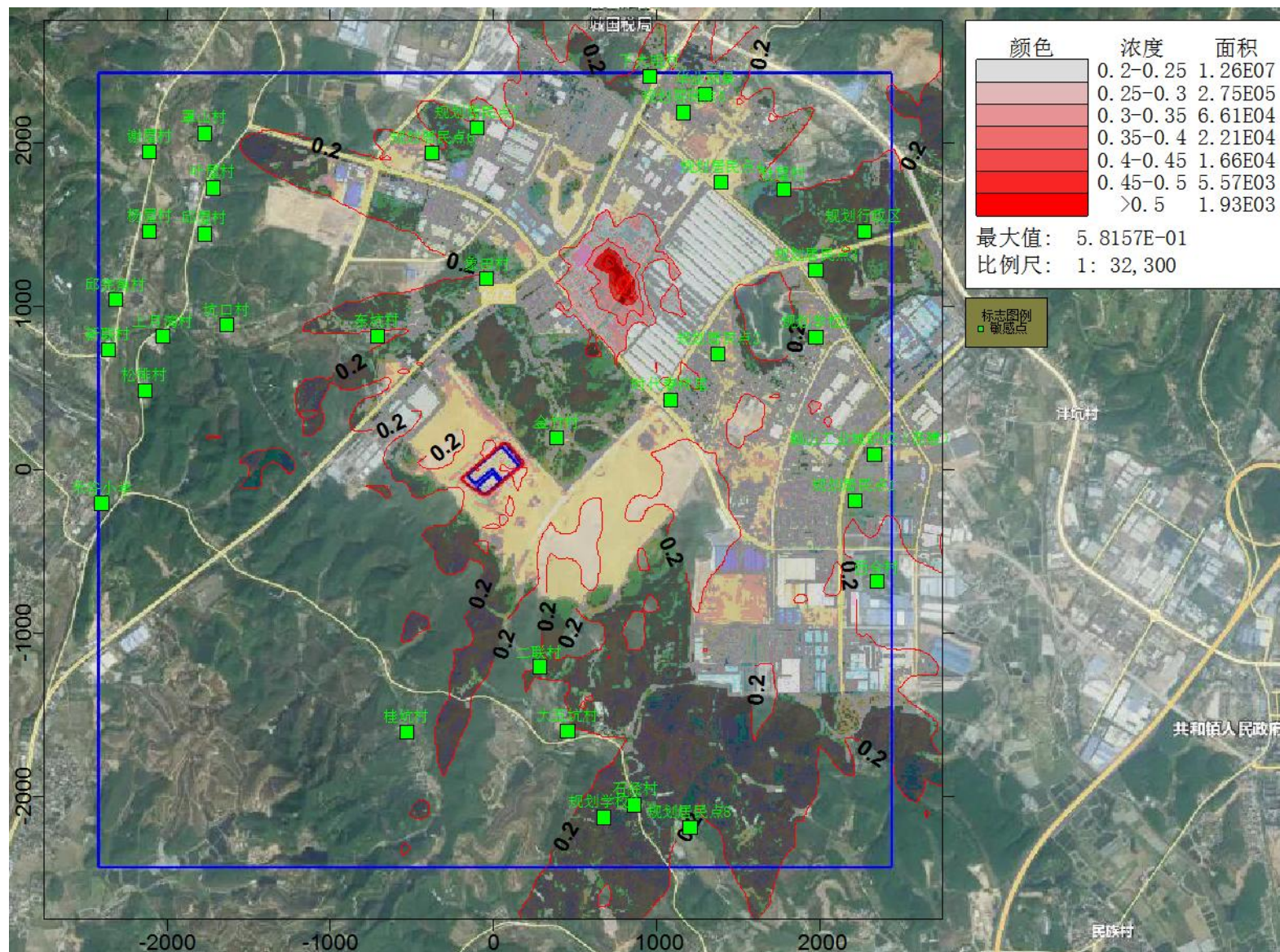
图 5.2-44 非甲烷总烃叠加区域在建拟建污染源和现状背景浓度小时质量浓度分布图
