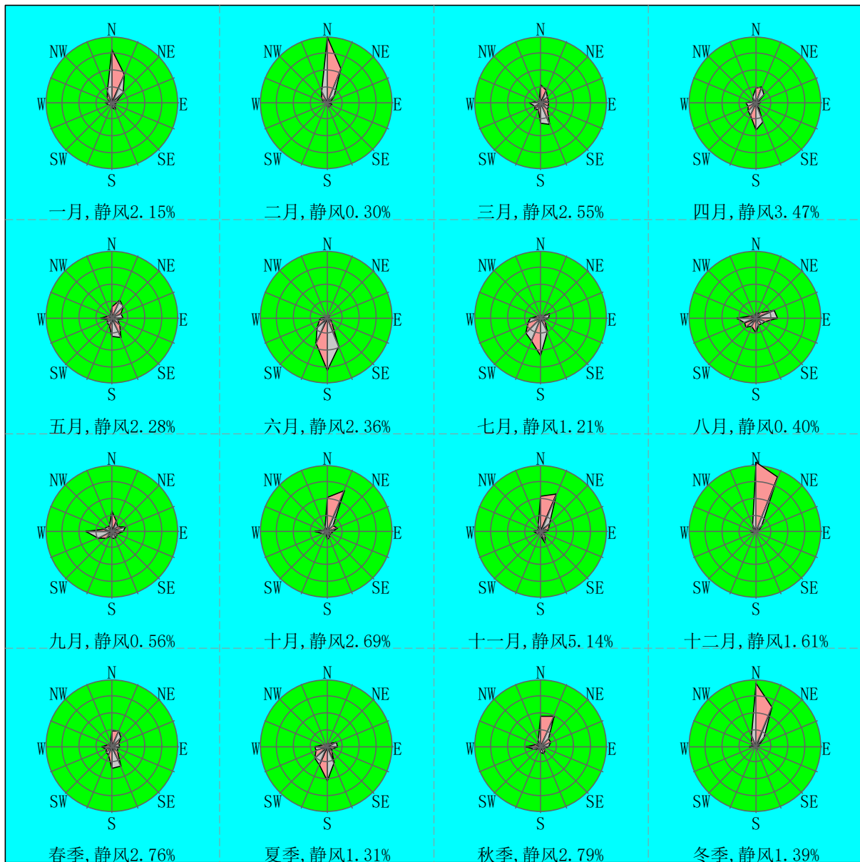
图 5.2-16 项目所在区域 2022 年各月及各季风频图
