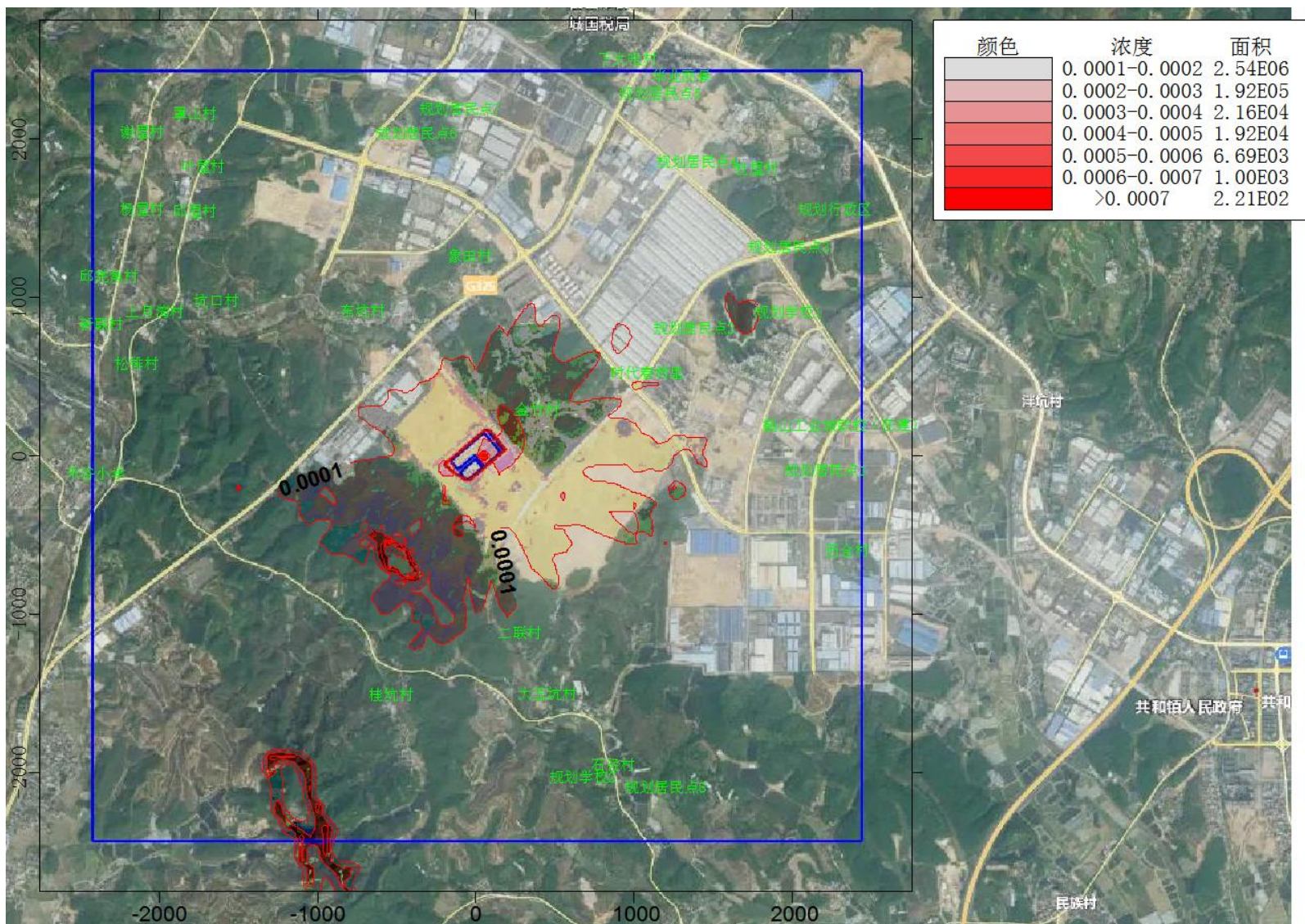
图 5.2-20 SO 2 新增污染源 1 小时平均贡献浓度分布图
