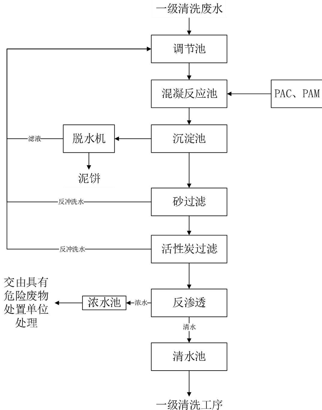
图 6.1-3 一级清洗废水处理工艺流程图
