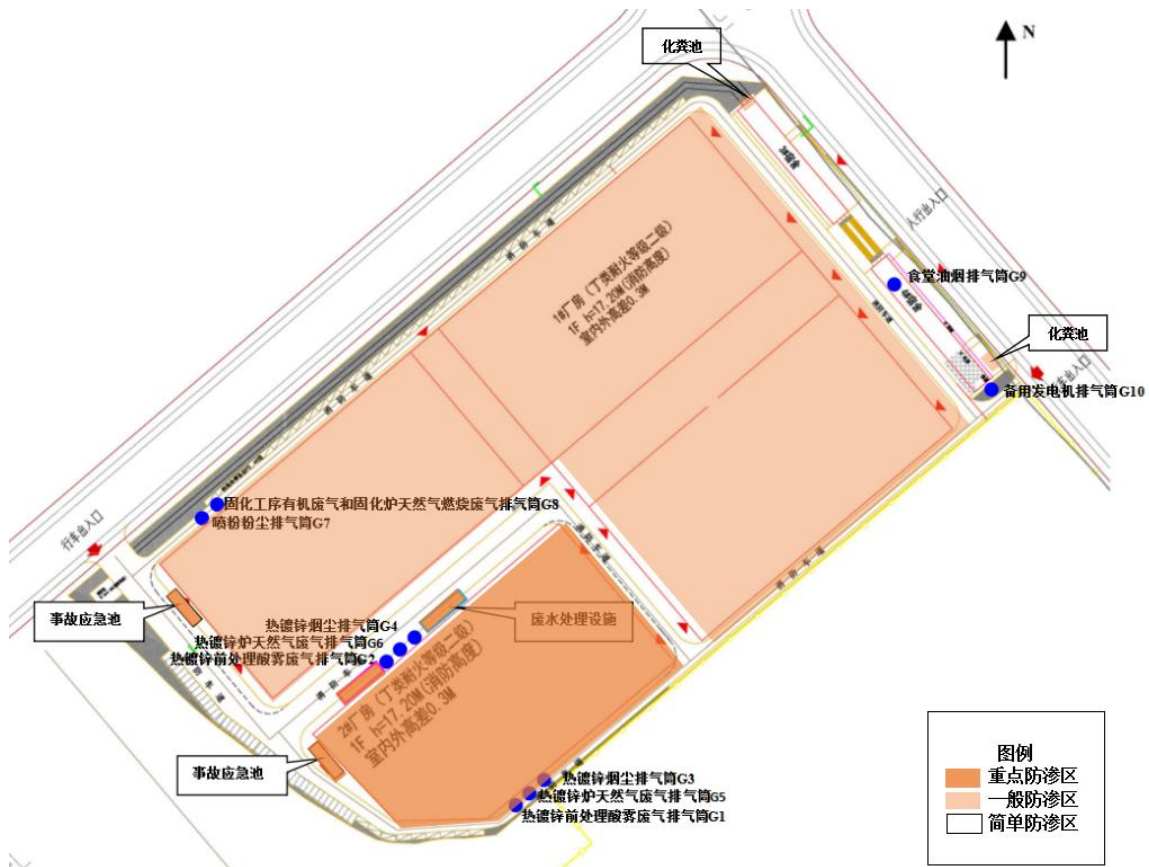
图6.1-3 本项目防渗分区图
