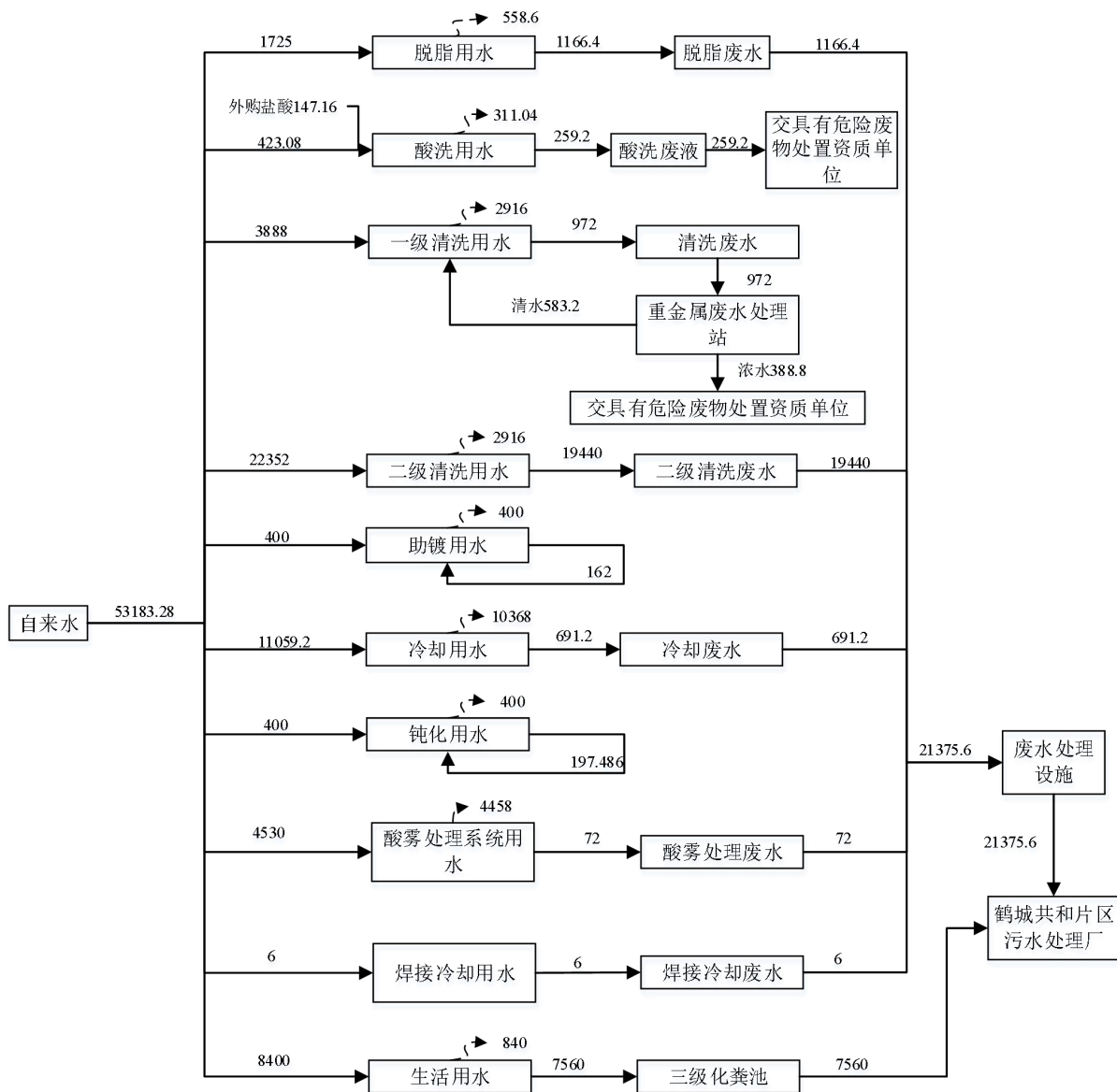
图 3.3-4 项目水平衡图 (单位 m^3/a )
