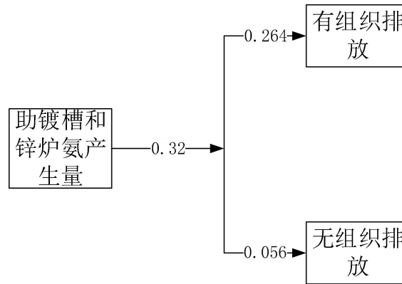
图3.3-3 本工程氨平衡图
