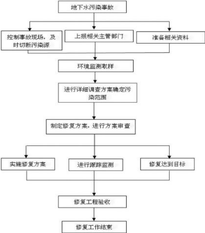
图6.1-6 地下水污染应急治理程序
