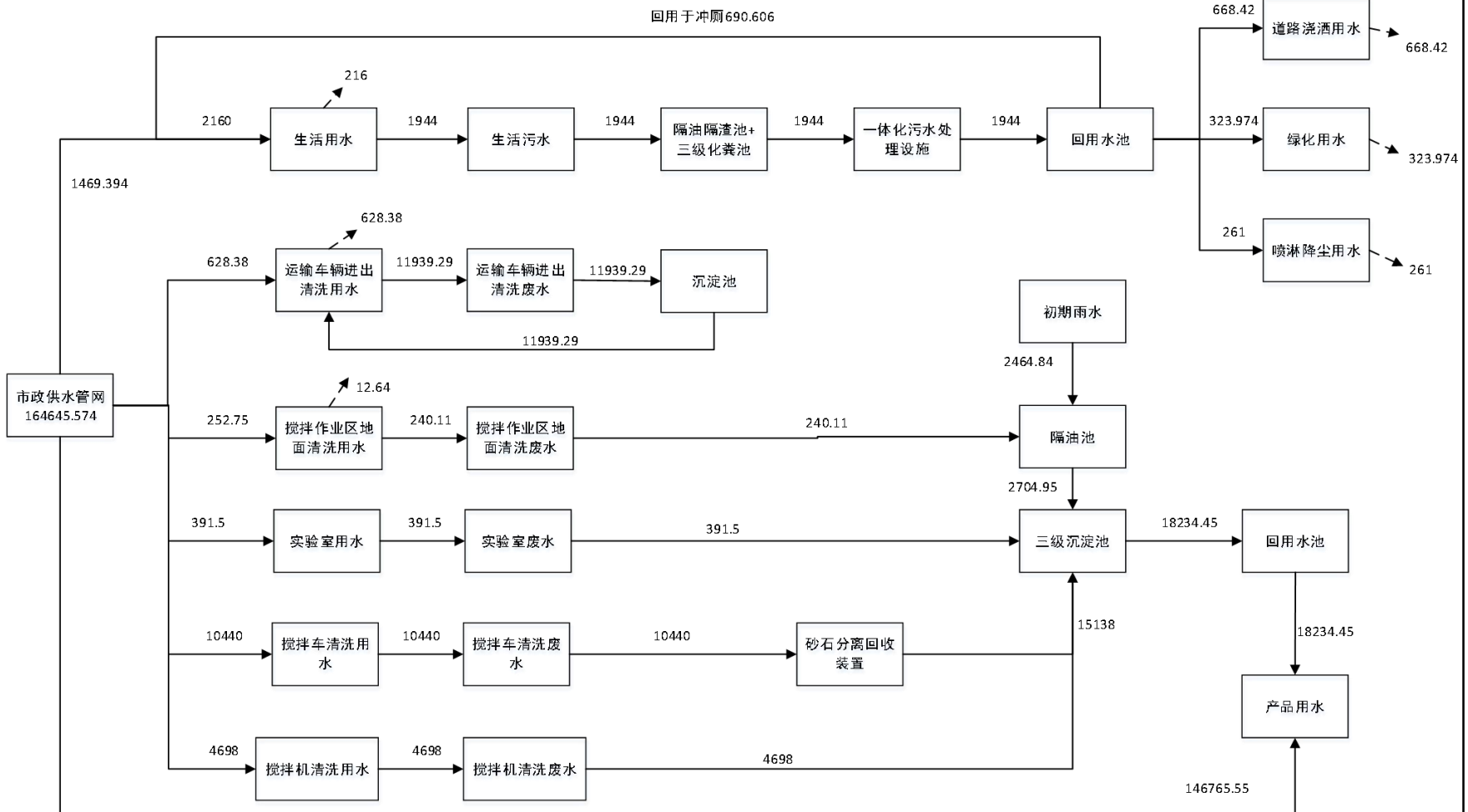
图 2-1 迁扩建后水平衡图 单位：m 3 /a
