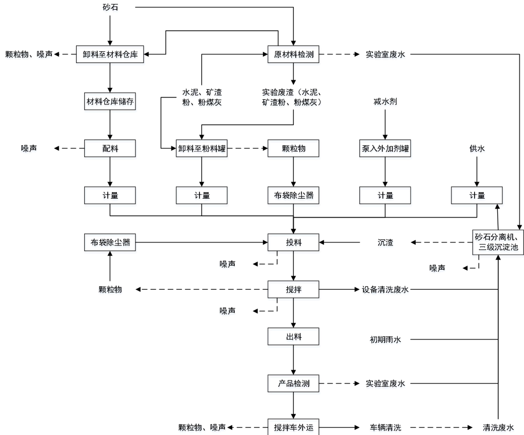
图 2-3 运营期工艺流程及产污环节简介图
