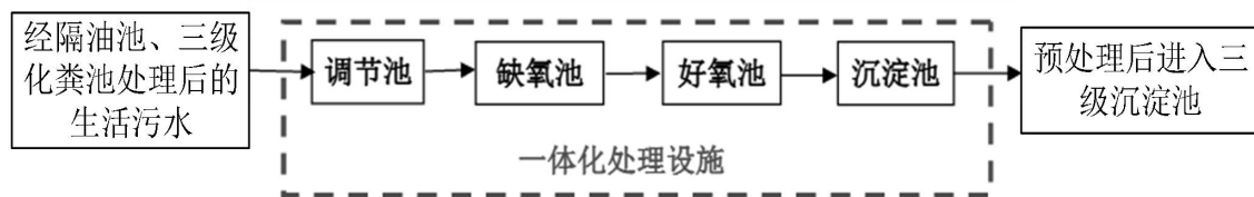
图4-1 一体化处理设施工艺流程图
