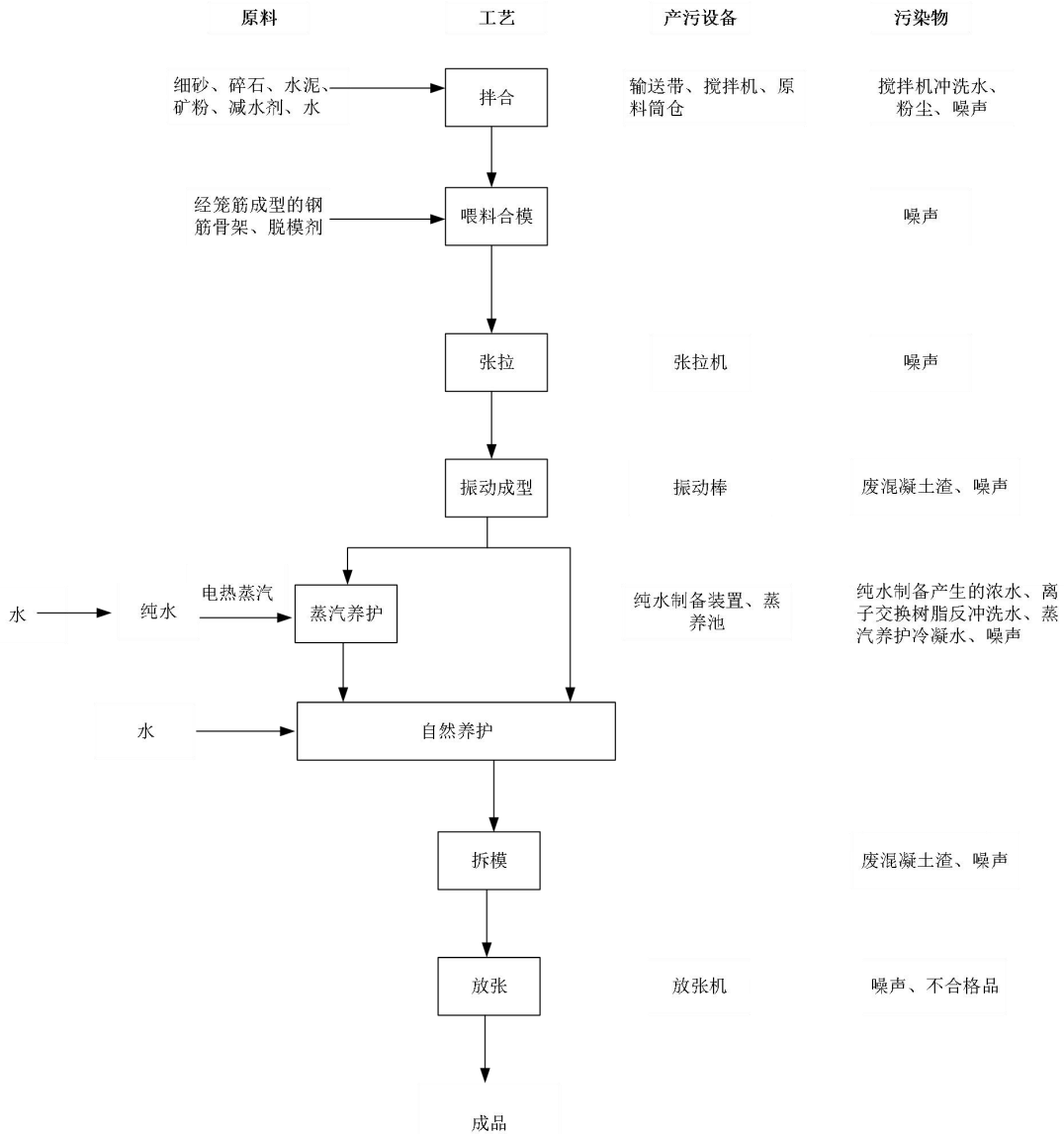
图 2-4 预应力混凝土方桩生产工艺流程图
