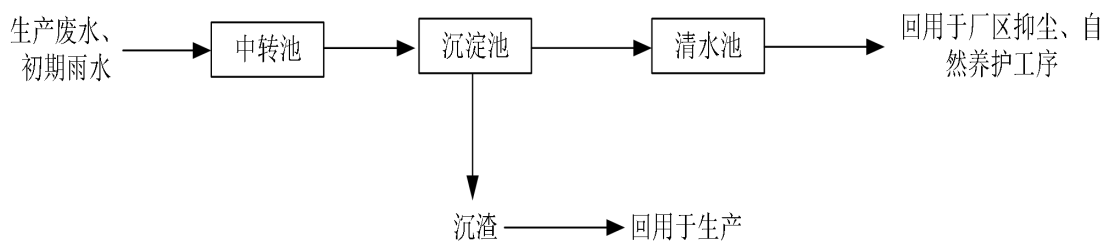
图4-2 废水处理设施工艺流程图
