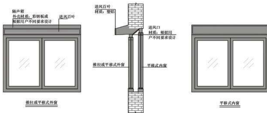
图 8.2-3 通风隔声窗示意图
