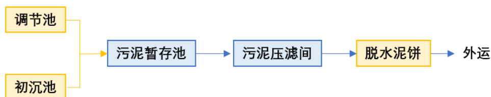
图 4.4-6 现有一期工程污泥处理工艺流程图
