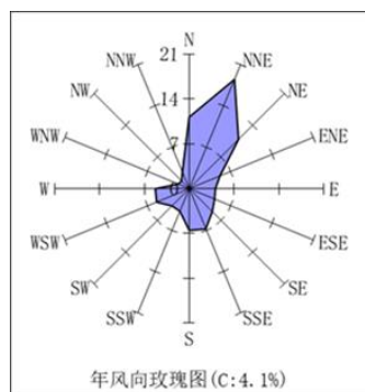
图 7.1-1 新会气象站累年年平均风向玫瑰图（统计年限：2001-2020 年）
