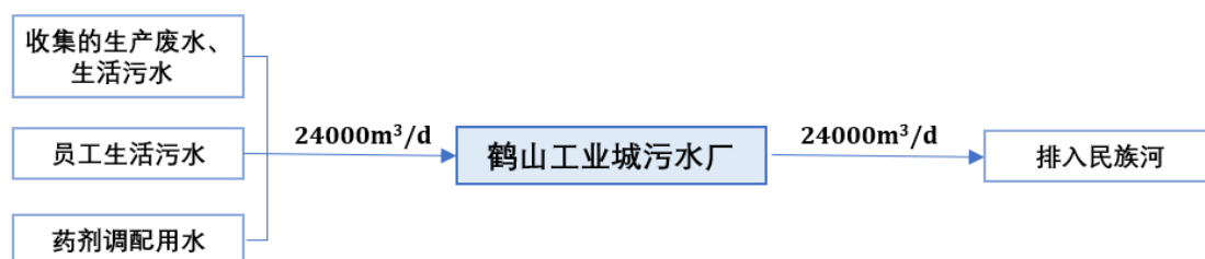
图 4.4-10 改扩后全厂水平衡图
