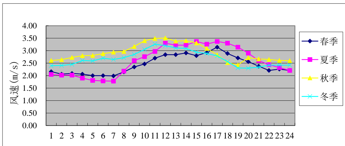
图 7.1-4 新会 2020 年平均风速月变化曲线图
