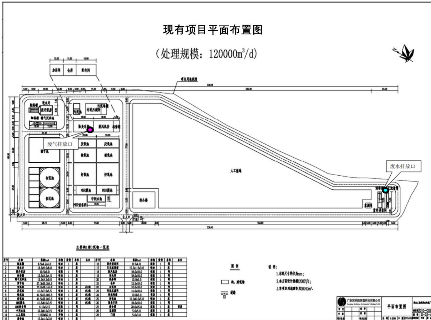
图 3.2-1 现有工程平面布置图
