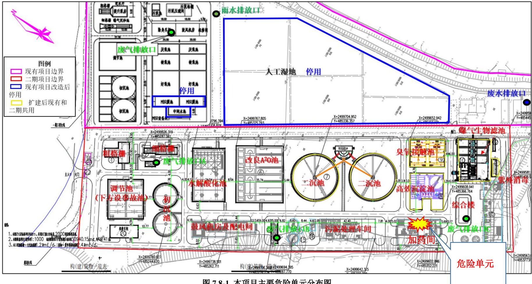
图 7.8-1 本项目主要危险单元分布图
