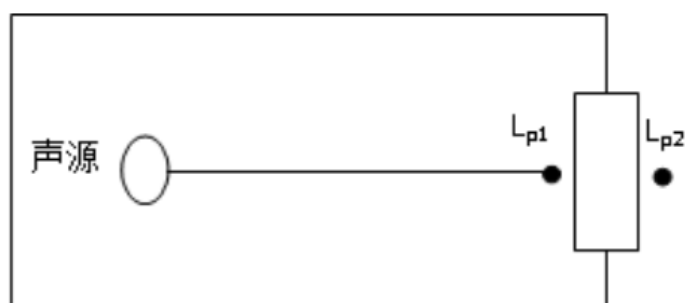
图 7.4-1 室内声源等效为室外声源图例
