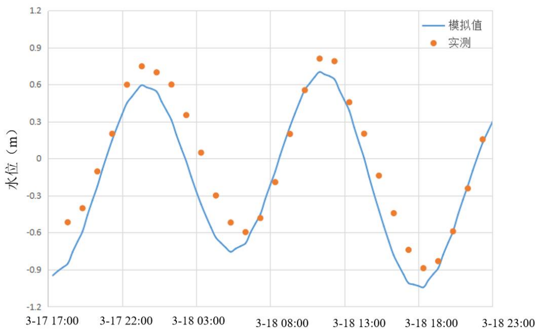
高栏岛水位验证-枯水期
