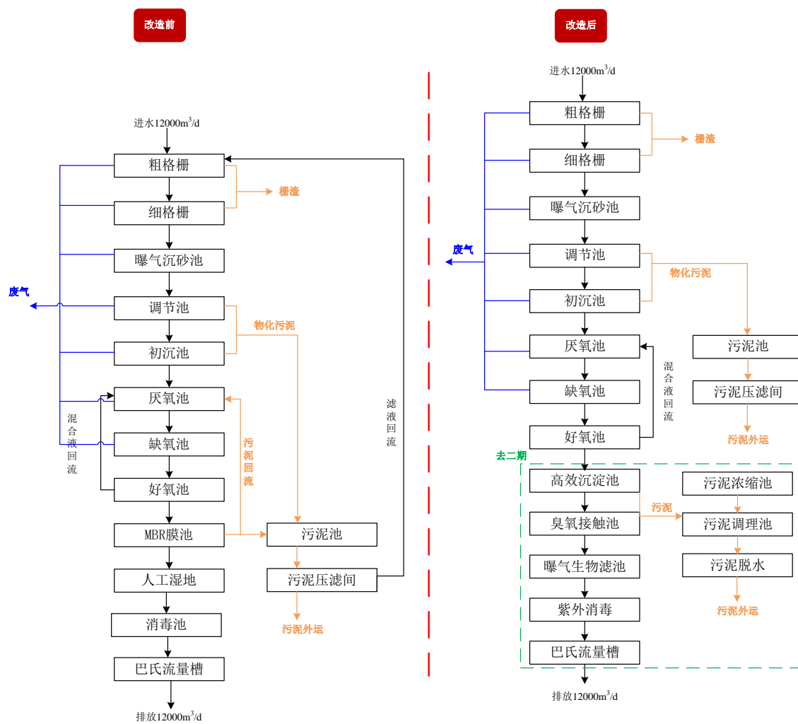
图 4.4-3 现有工程改造前后对比图
