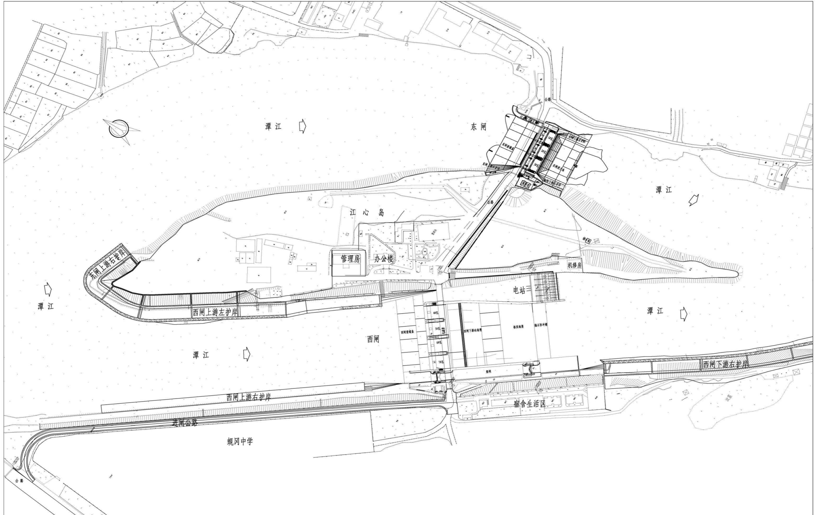
附图4 合山水电站平面布置图
