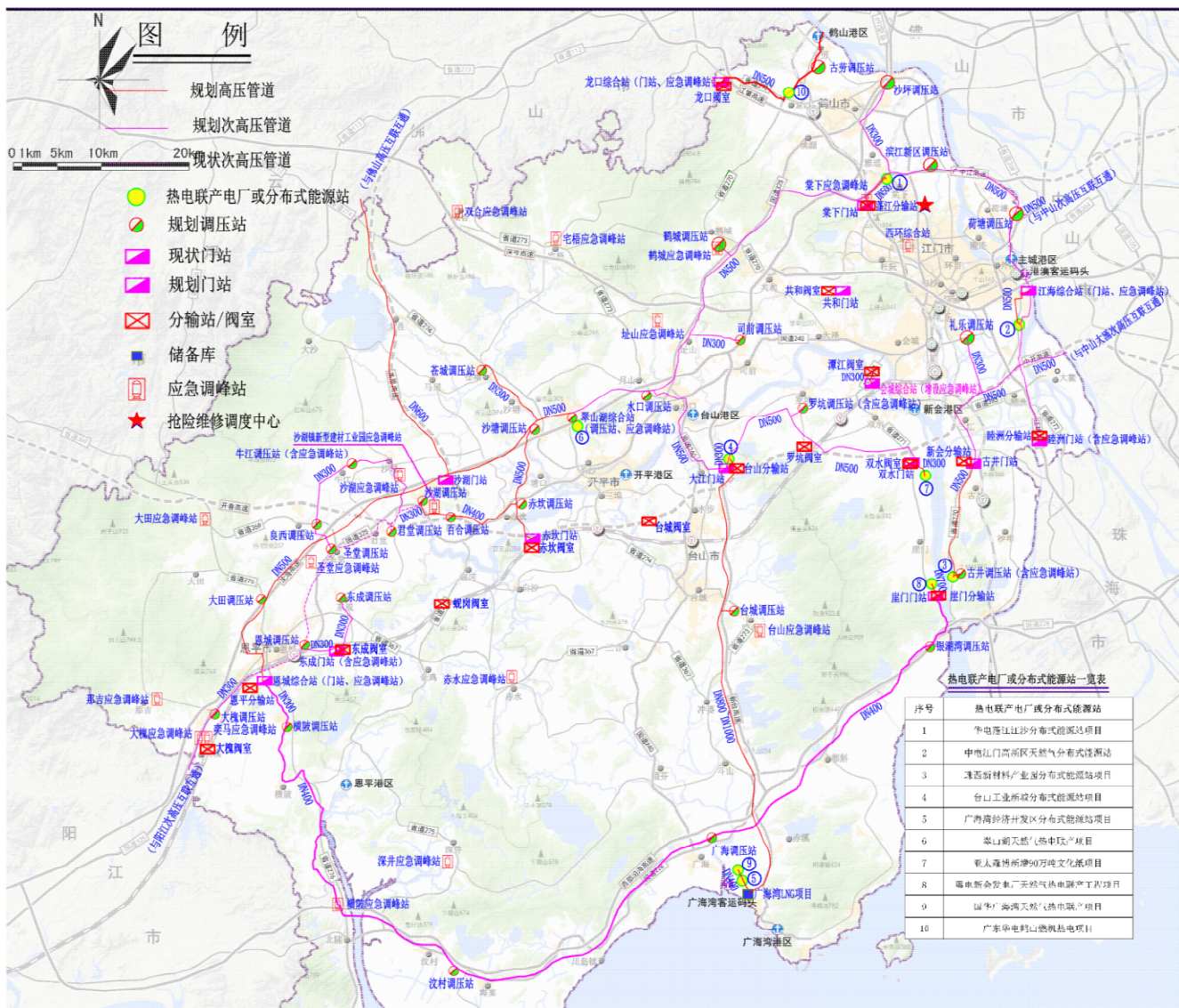
图 12 市域高压管道、市域次高压管道规划图
