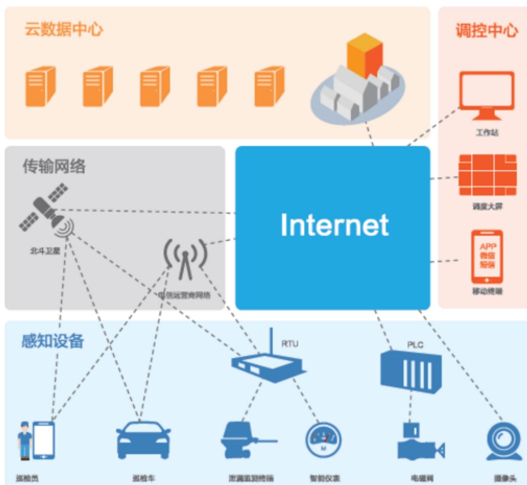
图 15 智慧燃气概览图
