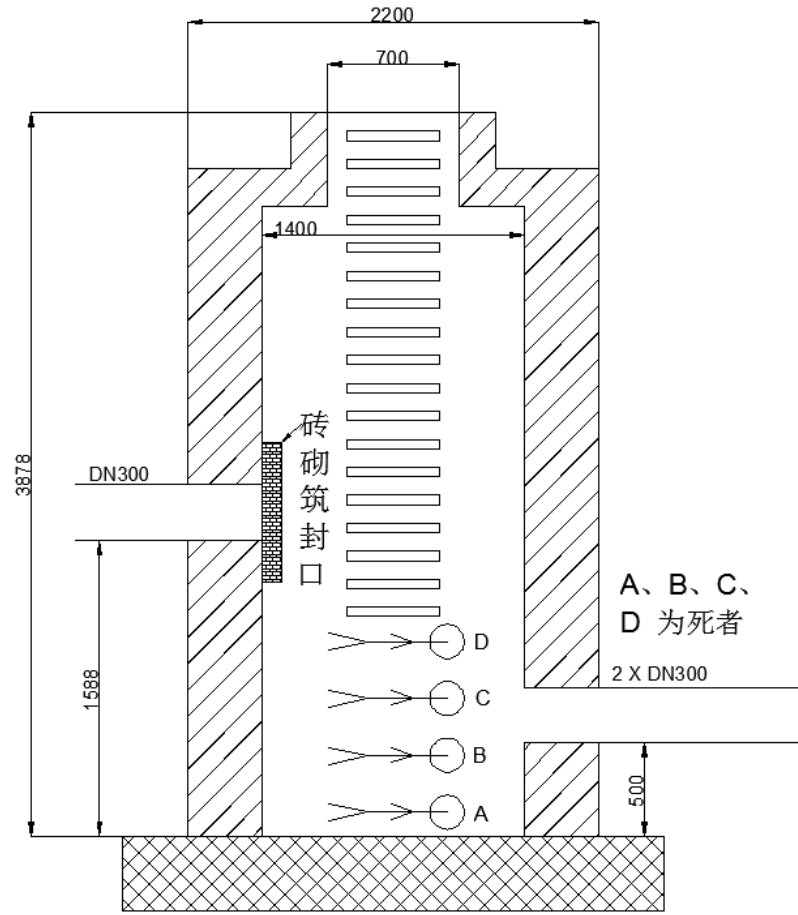
图2 A46#事故井示意图
